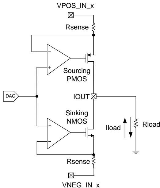
图 101. Current Output
