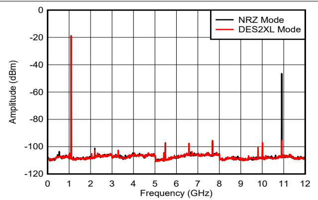
图 6-11. f_{\text{OUT}} = 1097\text{MHz} ， 0\text{dBFS}
