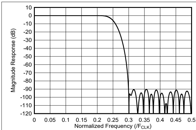
图 7-14. 2 倍内插滤波器响应
