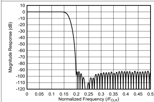
图 7-16. 3 倍内插滤波器响应
