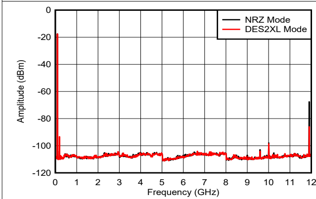
图 6-8. f_{\text{OUT}} = 97\text{MHz} ， 0\text{dBFS}
