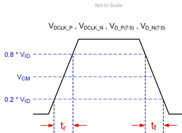
图 5-5. SubLVDS 输入上升和下降压摆率
