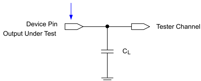
图 5-14. 输出传播测量的测试负载电路
