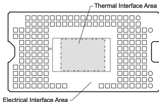
图 5-15. 系统安装接口负载
