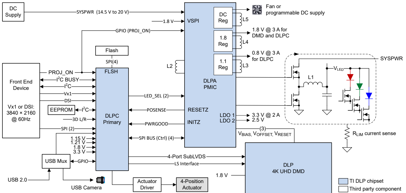
图 7-1. 典型 4K 超高清 LED 应用图
