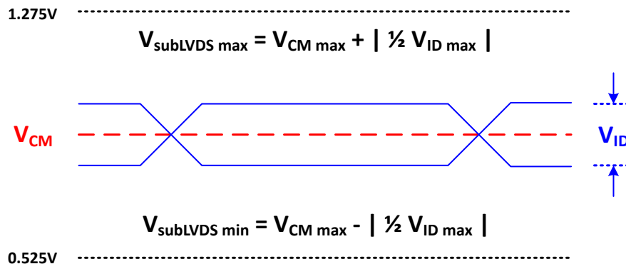
图 5-10. SubLVDS 波形参数
