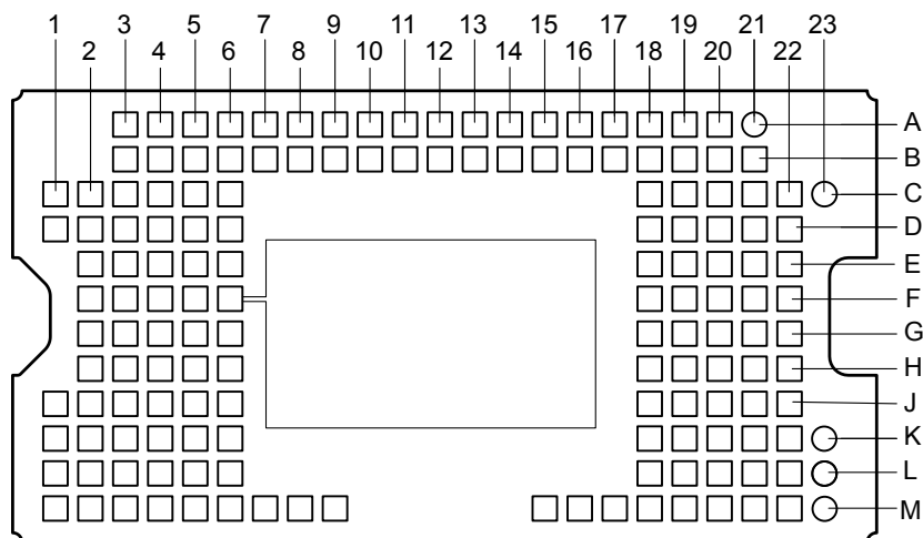
图 4-1. FSB 封装，154 引脚 LGA (底视图)
