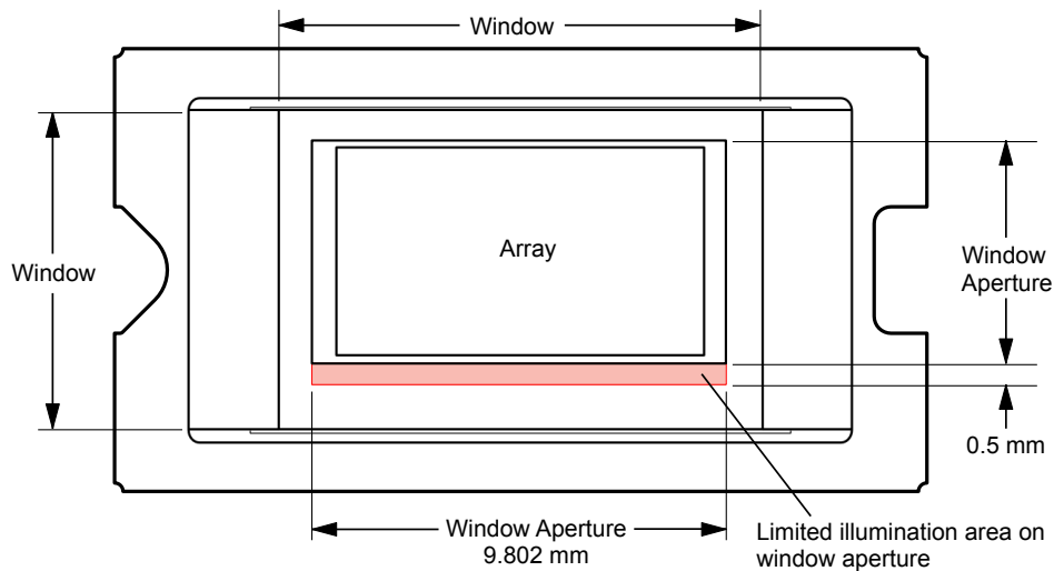
图 5-2. 照明溢出图 — 关键区域
