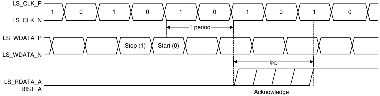
图 5-3. 开关特性
