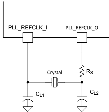
图 9-1. 晶体所需的分立式元件
