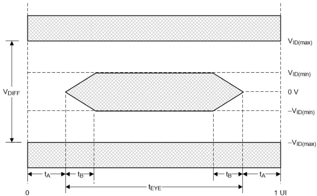
图 6-8. V-By-One 时序
