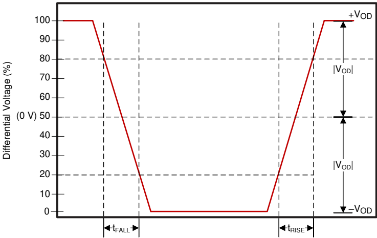
图 6-3. 差分输出信号
