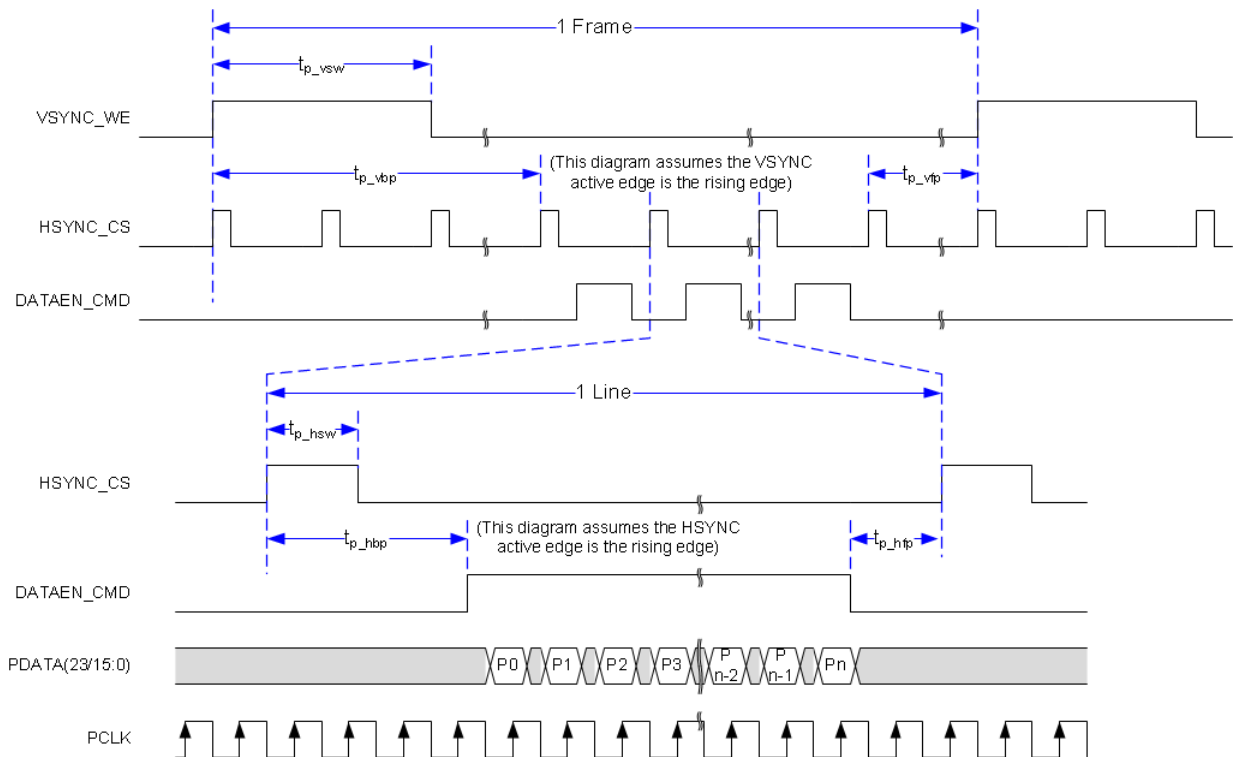
图 6-10. 源帧时序
