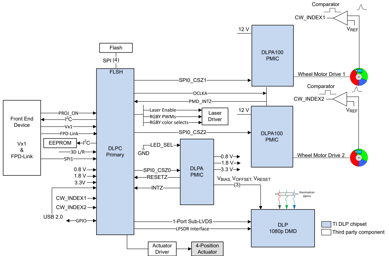
图 7-2. 激光荧光功能方框图
