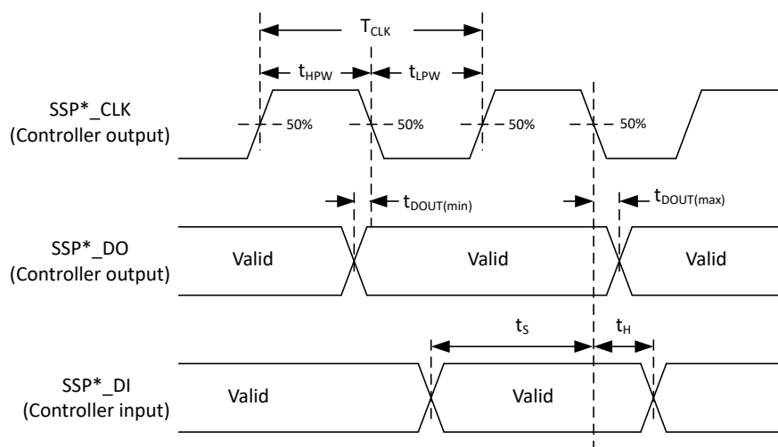
图 6-12. SSP 主机模式 (模式 0/3) 的时序图
