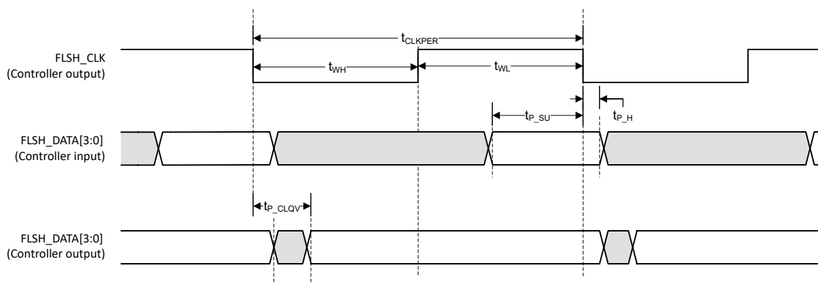
图 6-9. 闪存接口时序
