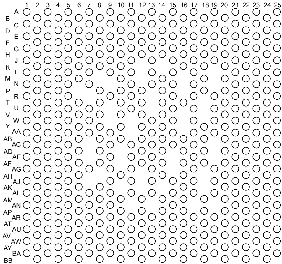
图 5-1. AMD 封装 484 引脚 FCCSP 顶视图
