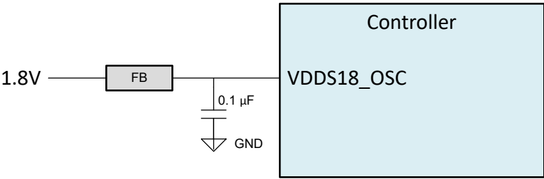
图 9-2. 晶体电源滤波
