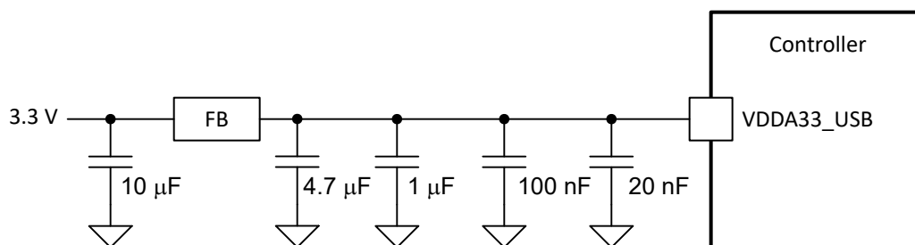
图 9-5. VDDA33_USB (USB) 推荐的滤波器
