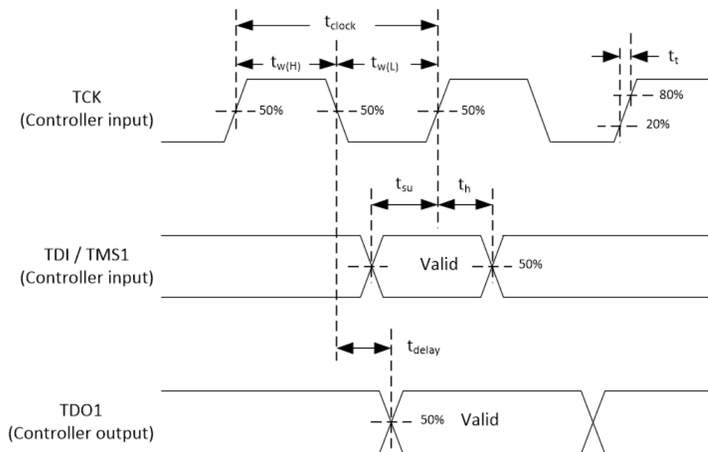
图 6-14. JTAG 边界扫描的时序图
