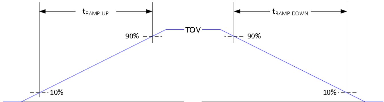
图 6-7. 电源斜坡时间
