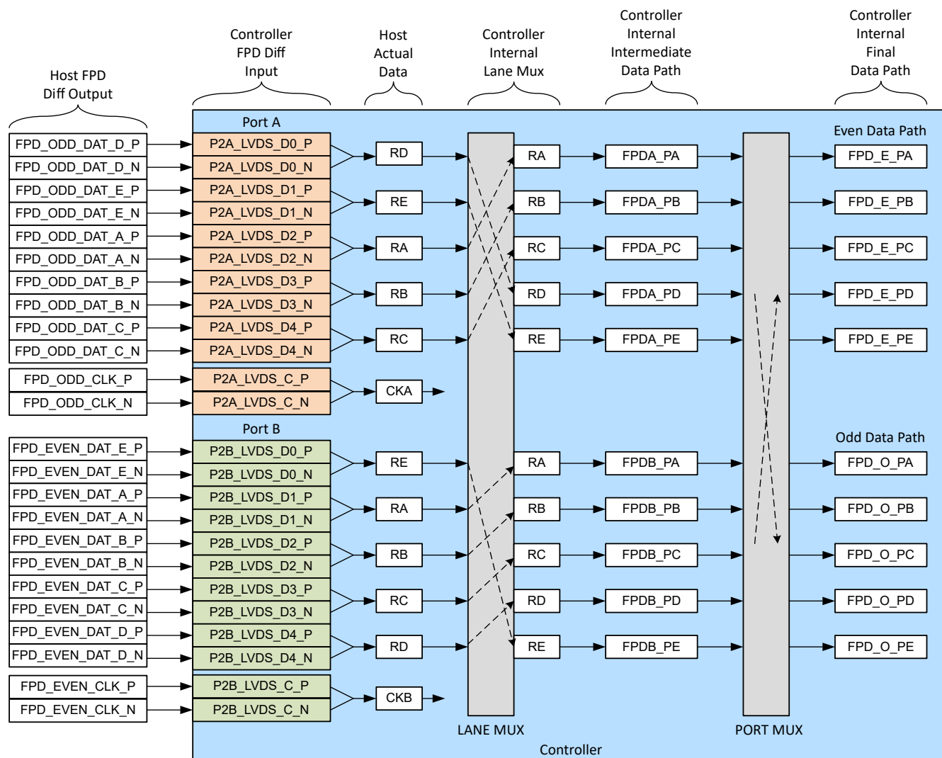
图 7-4. 备用 FPD-Link 端口通道映射示例
