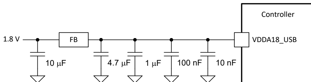
图 9-6. VDDA18_USB (USB) 推荐的滤波器
