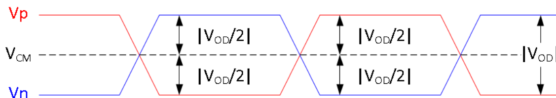
图 6-4. DMD 低速差分电压参数
