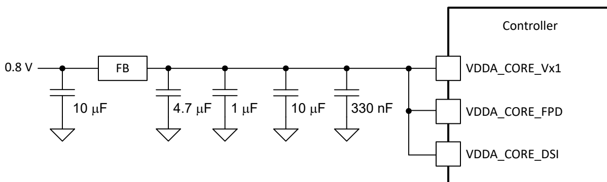
图 9-7. 针对 VDD_CORE_VX1 (V-by-One)、VDD_CORE_FPD (FPD-Link)、VDD_CORE_DSI (DSI) 建议的滤波器
