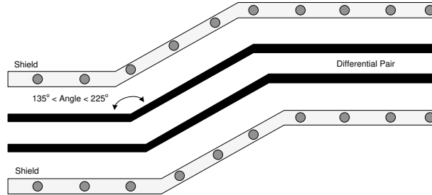
图 9-3. V-By-One 布线示例
