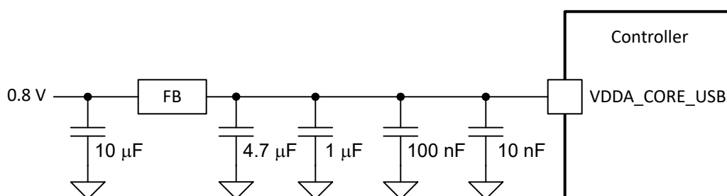
图 9-8. 针对 VDD_CORE_USB (USB) 建议的滤波器
