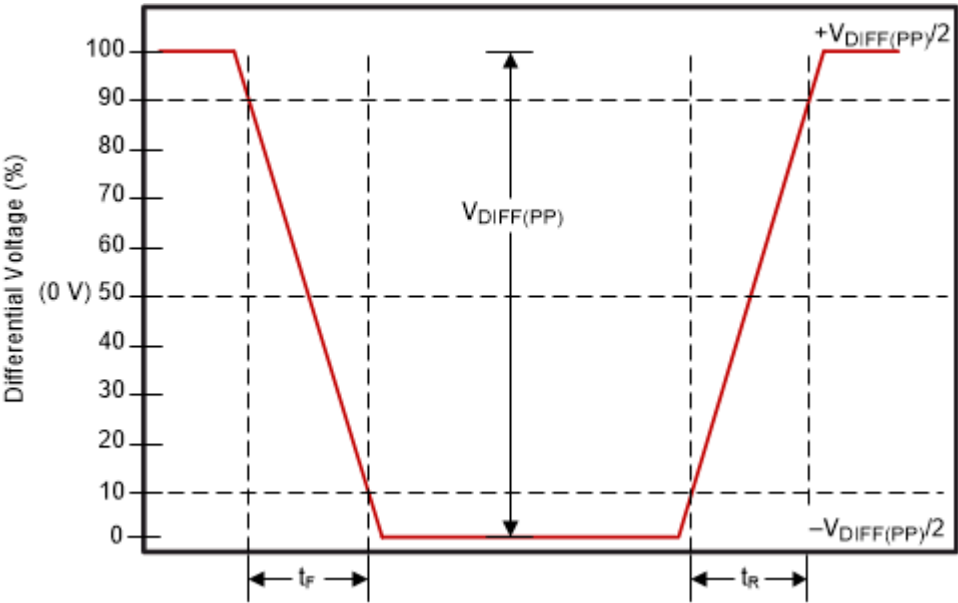
图 6-15. DMD 低速差分时序参数
