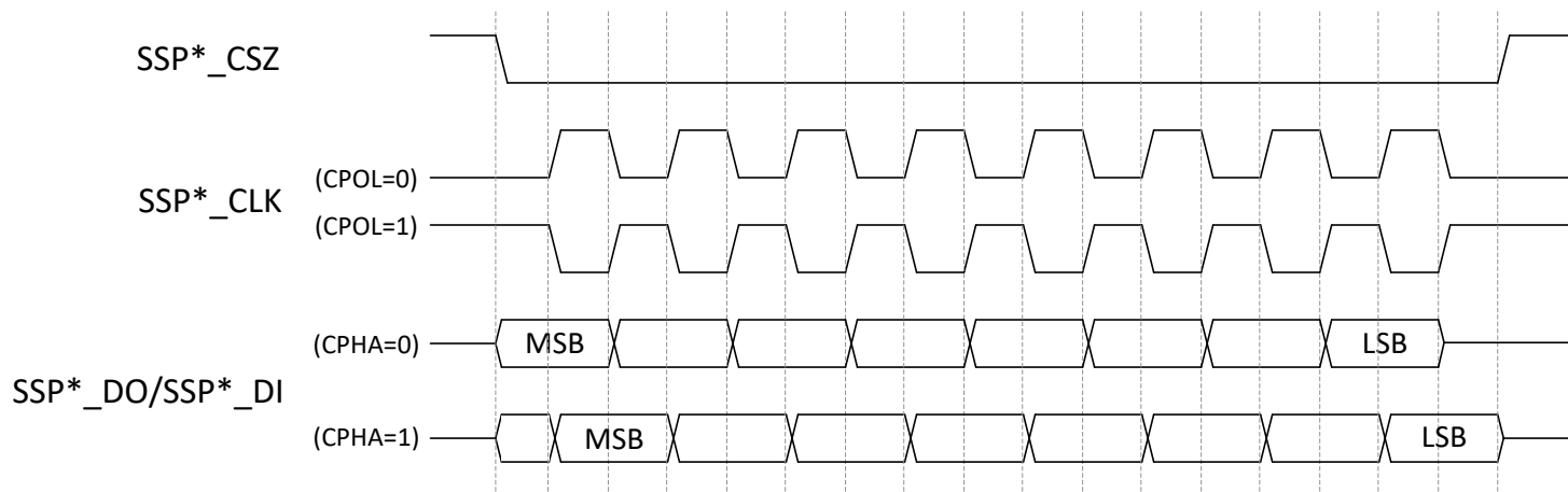
图 6-11. SPI 时钟模式的时序图
