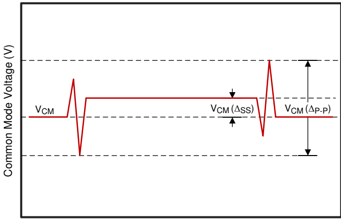
图 6-2. 共模电压
