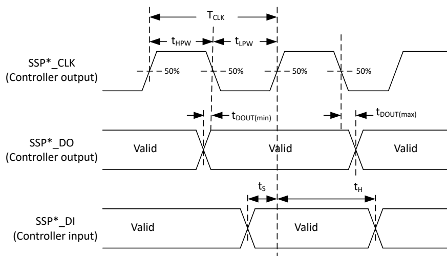
图 6-13. SSP 目标模式 (模式 0/3) 的时序图
