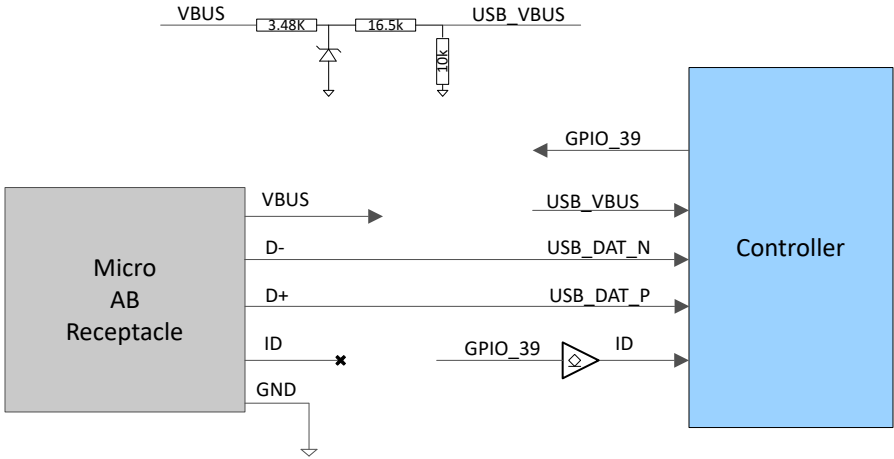
图 6-5. DLPC84x4 控制器的 USB 示例
