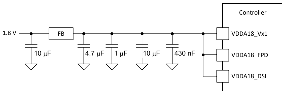
图 9-4. 针对 VDDA18_VX1 (V-by-One)、VDDA18_FPD (FPD-Link)、VDDA18_DSI (DSI) 建议的滤波器
