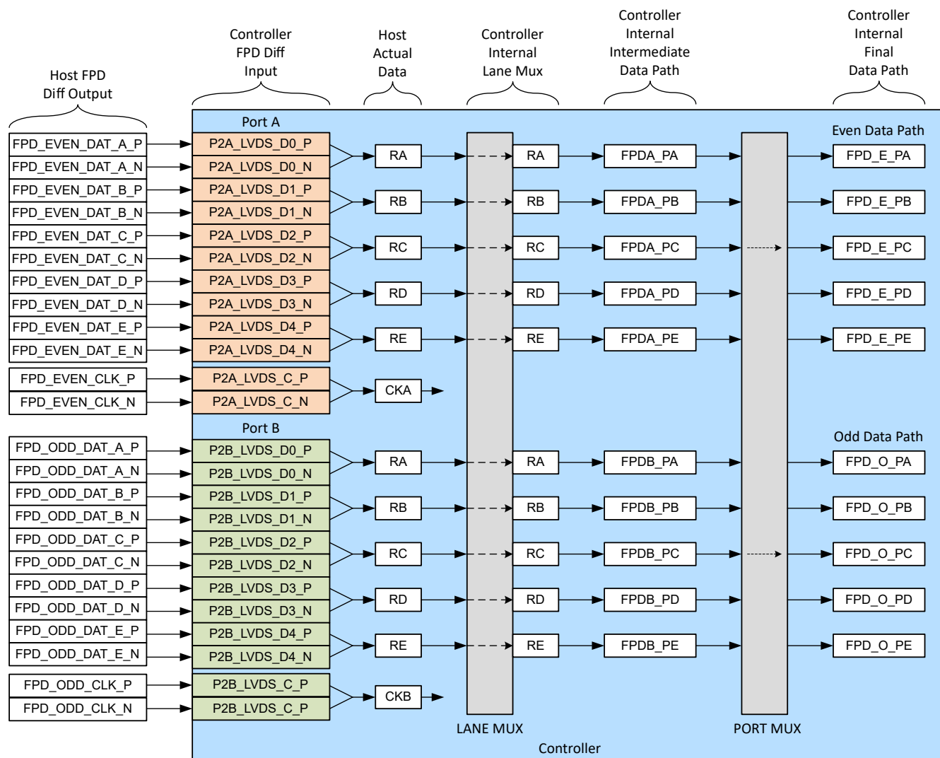
图 7-3. 典型 FPD-Link 端口通道映射示例
