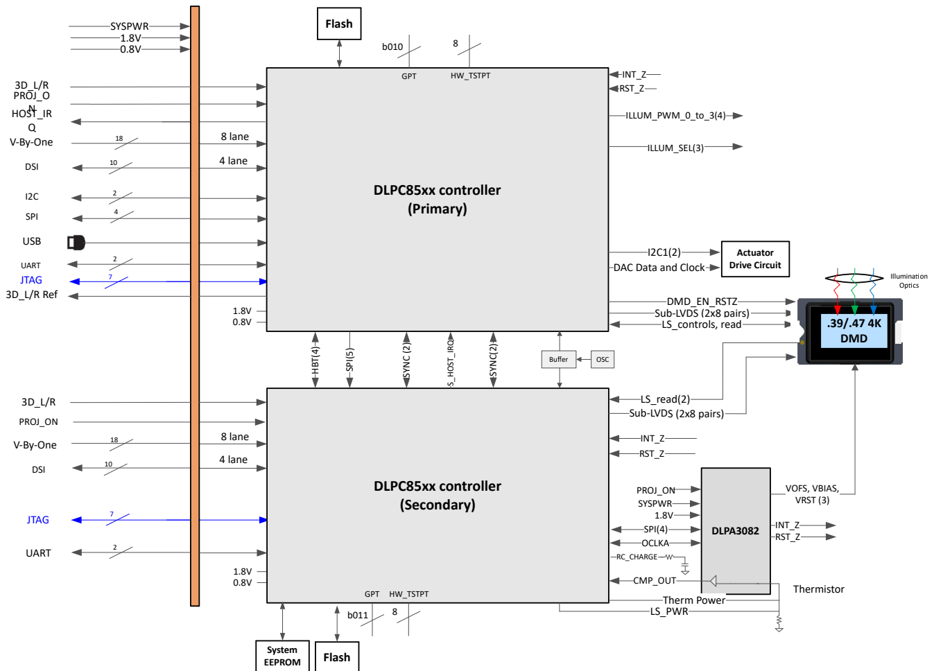
图 6-1. LED 和 RGB 激光功能方框图
