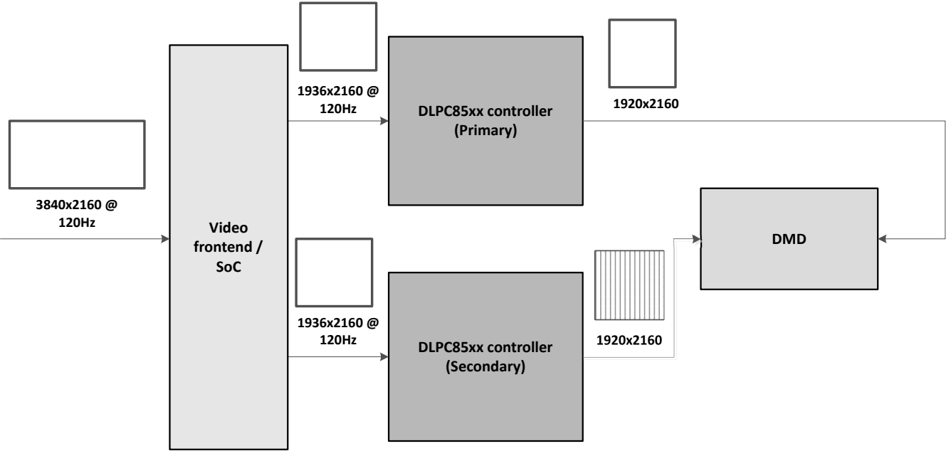
图 6-2. 具有视频输入分辨率的系统方框图
