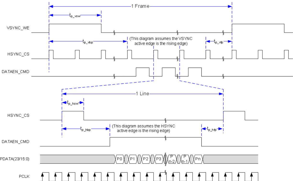
图 5-10. 源帧时序
