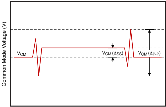
图 5-2. 共模电压
