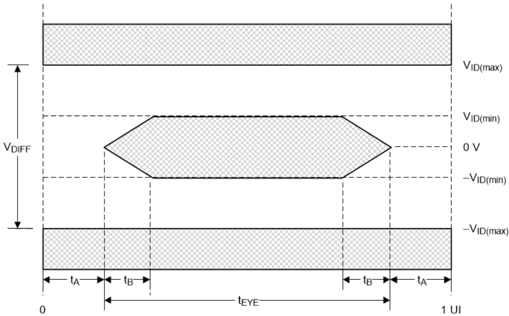
图 5-8. V-By-One 时序
