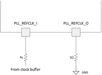
图 8-1. 时钟振荡器所需的分立式元件
