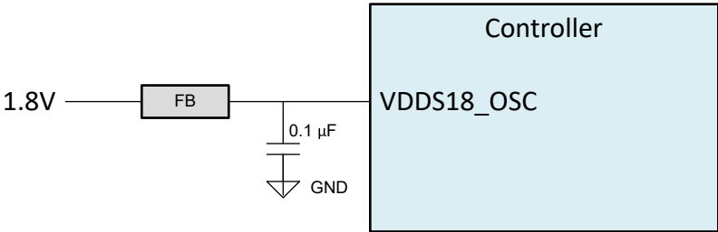
图 8-2. 时钟振荡器电源滤波
