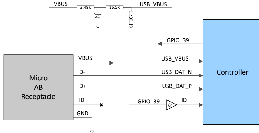
图 5-5. DLPC8545 控制器的 USB 示例
