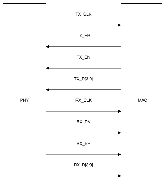
图 7-10. MII Signaling
