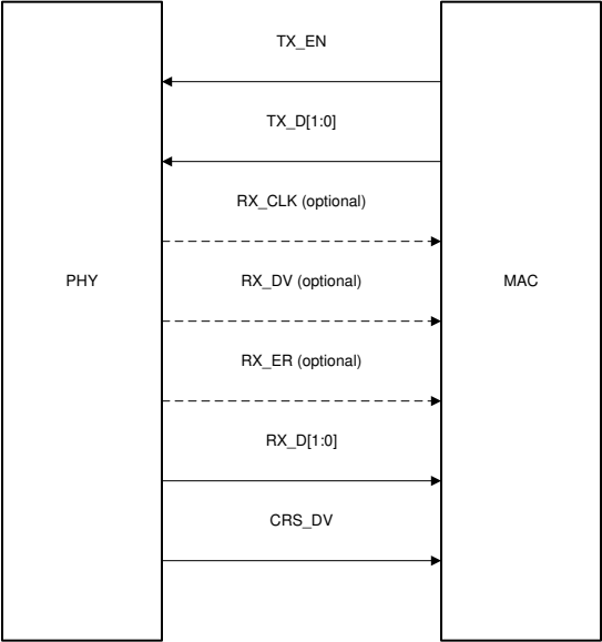
图 7-12. RMII 信令
