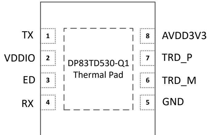
图 5-1. DP83TD530-Q1 引脚排列 (顶视图)
