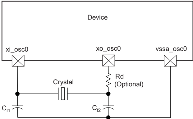
图 6-2. Crystal Implementation
