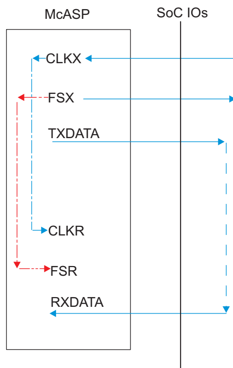
图 7-48. McASP1-8 CI-FO- – SYNC Mode
