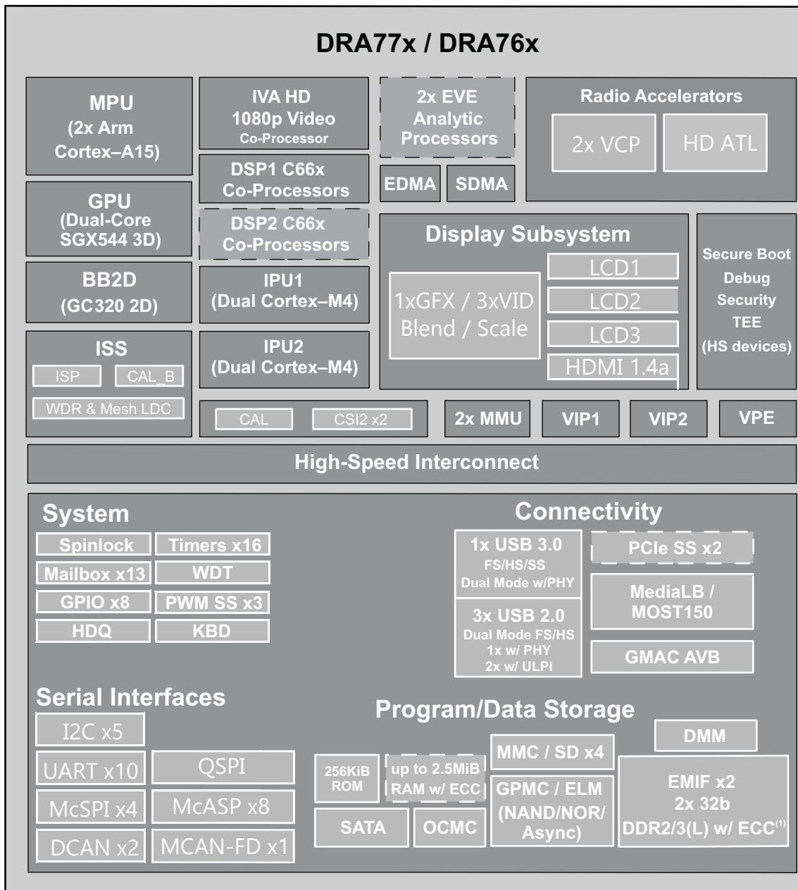
图 1-1. DRA77xP、DRA76xP 方框图
