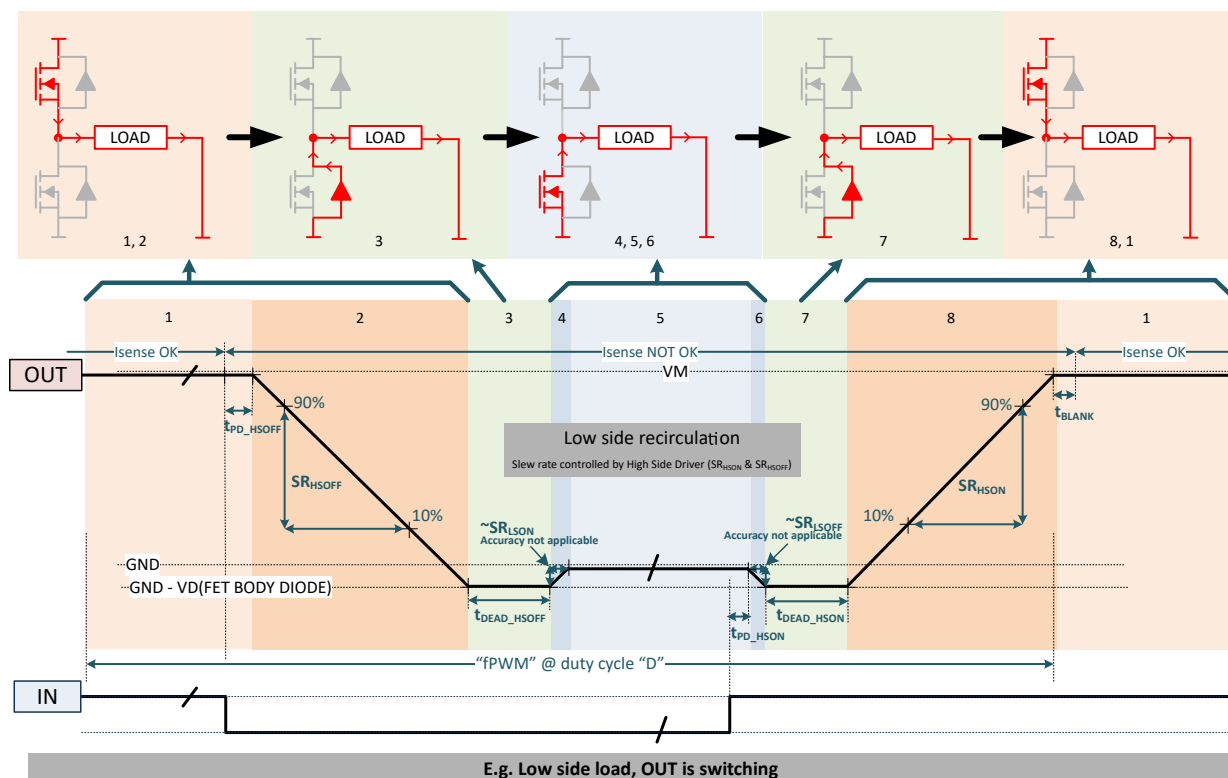
图 6-3. 具有低侧再循环的输出开关瞬态
