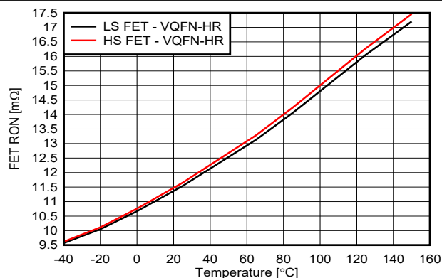
图 6-10. V_{VM} = 13.5V 时 R_{HS\_ON} 和 R_{LS\_ON} 与温度之间的关系
