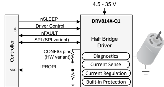
简化原理图
