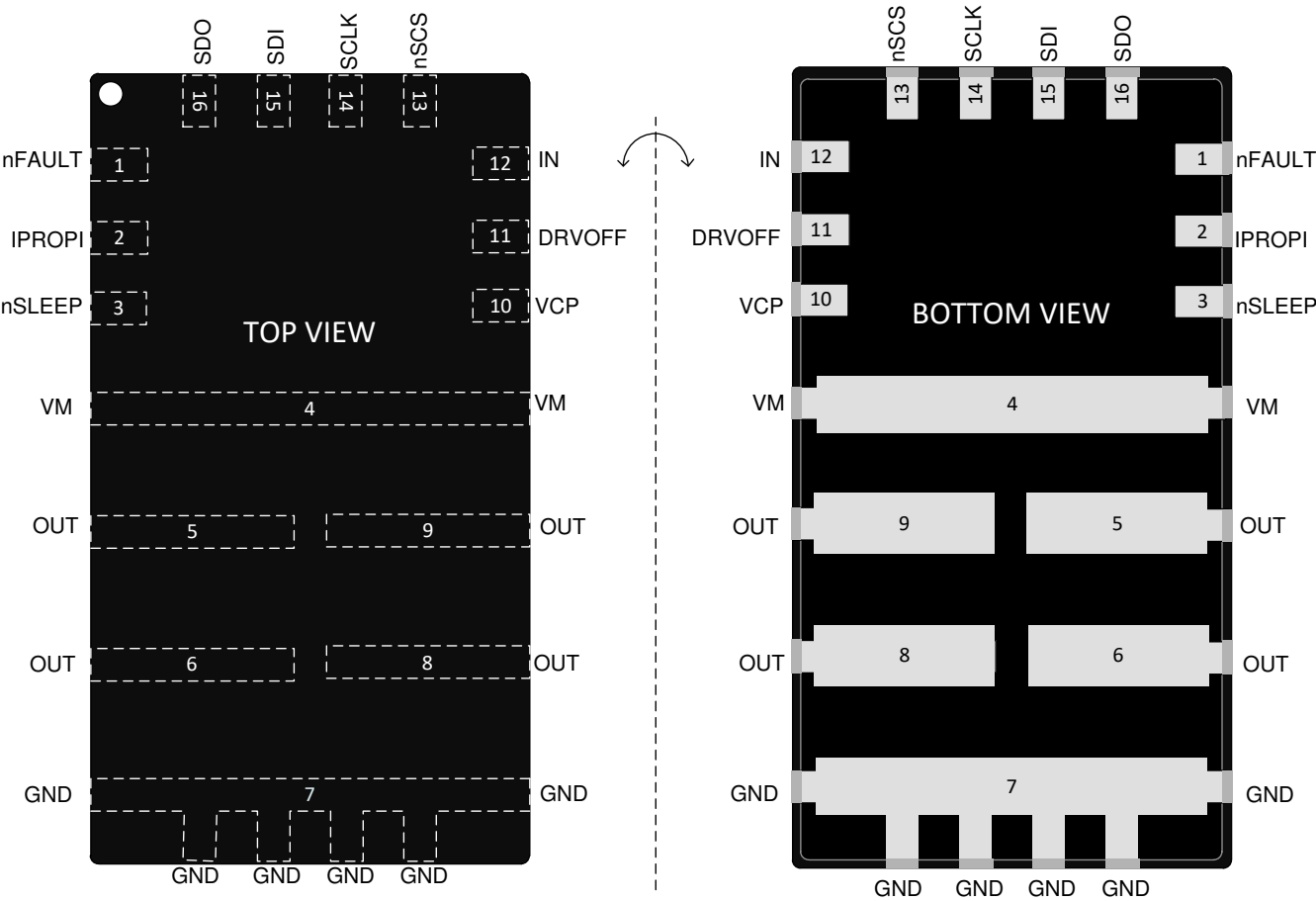
图 5-2. 采用 VQFN-HR (16) 封装的 DRV8144S-Q1 SPI 型号
