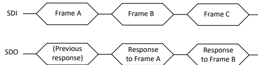
图 7-20. SPI 通信期间 SDI 和 SDO 之间的关系
