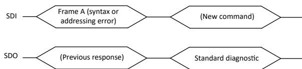
图 7-24. 命令语法错误后的响应
