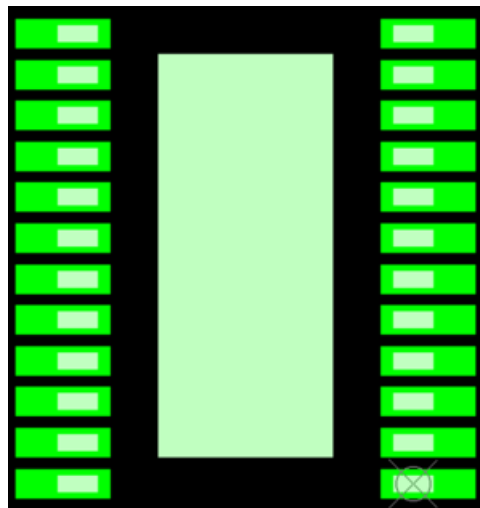
图 8-2. PWP0024T PCB 焊盘上的 SO-24，白色：其他 SO-24 引线，绿色：TI PWP0024T PCB 焊盘
