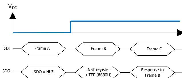
图 7-23. 退出 V DD 上电复位后的响应
