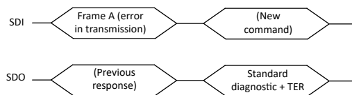
图 7-22. 传输出错之后的响应
