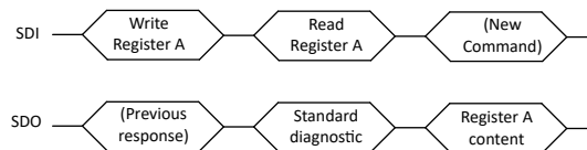
图 7-21. 寄存器内容发送回微控制器
