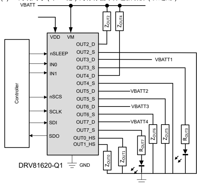
图 3-1. 简化版原理图
