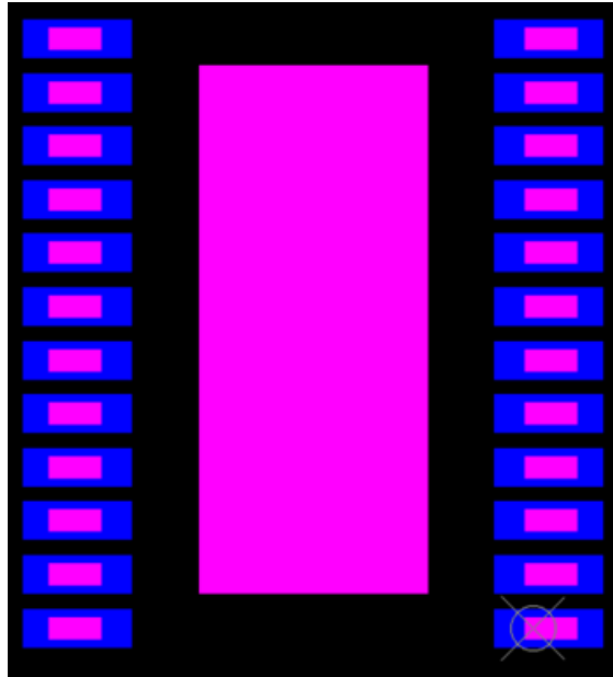
图 8-1. 另一 SO-24 PCB 焊盘上的 PWP0024T，粉色：TI PWP0024T 引线，蓝色：其他 SO-24 PCB 焊盘
