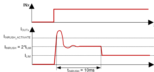
图 6-15. 浪涌期间的电流限制值
