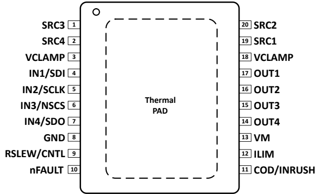
图 4-1. 20 引脚 PWP 封装 HTSSOP (顶视图)
