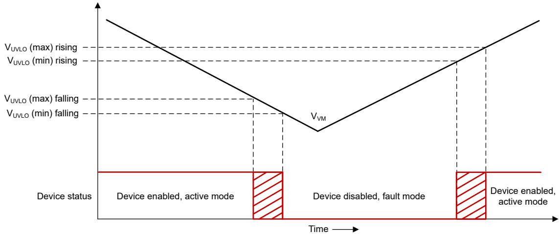
图 6-17. VM UVLO 运行
