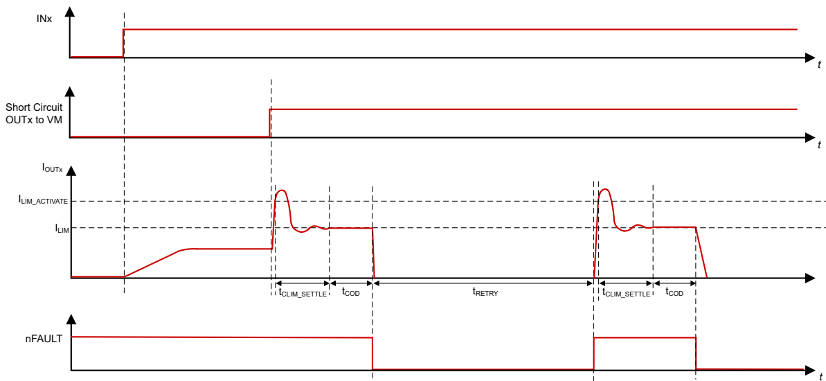
图 6-14. 启用 COD 时的电流限制电路对短路的响应
