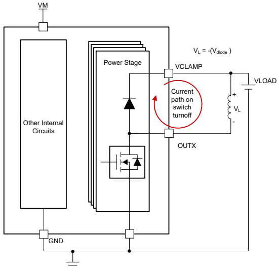
图 6-6. 慢速衰减 ( VCLAMP 连接至 VLOAD )
