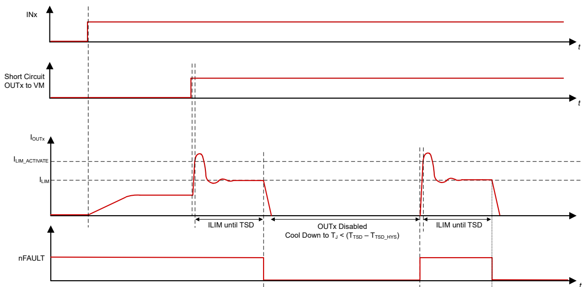
图 6-12. 在基于热关断的重试模式下对短路的电流限制响应 (截止延迟已禁用)
