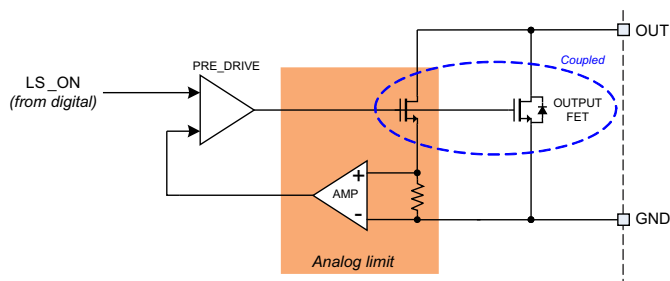
图 6-13. 模拟电流限制和检测图
