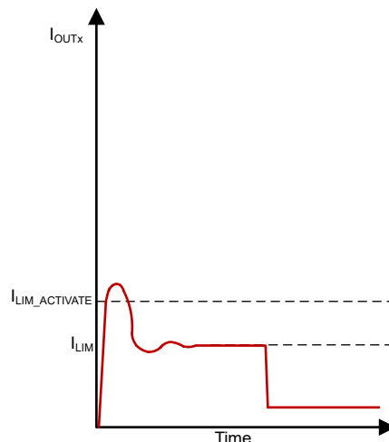
图 6-11. 浪涌电流，具有 ILIM 保护
