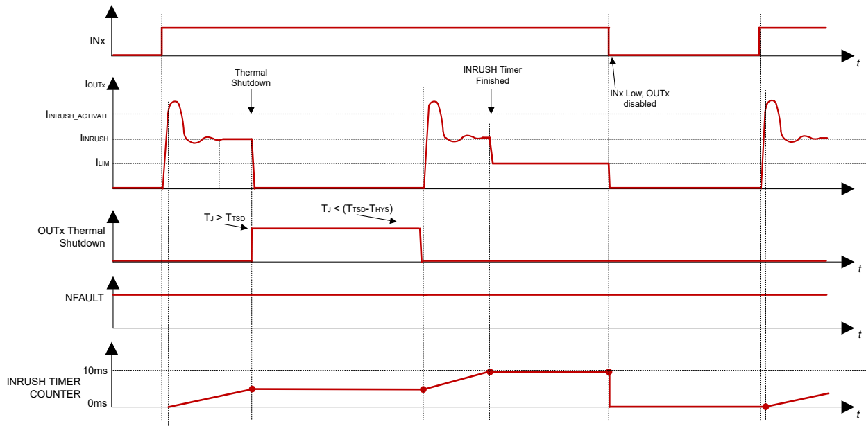
图 6-16. t_{\text{INRUSH}} 期间通道热关断的浪涌计时器示例
