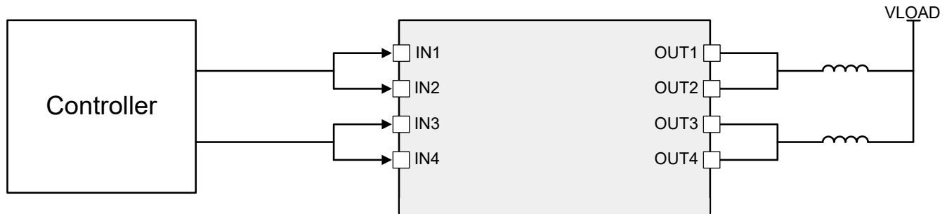
图 6-9. 以更高的电流驱动两个螺线管
