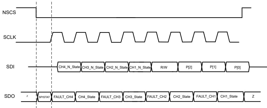
图 6-3. SPI 数据 - 标准“8 位”帧和 SPISTAT
