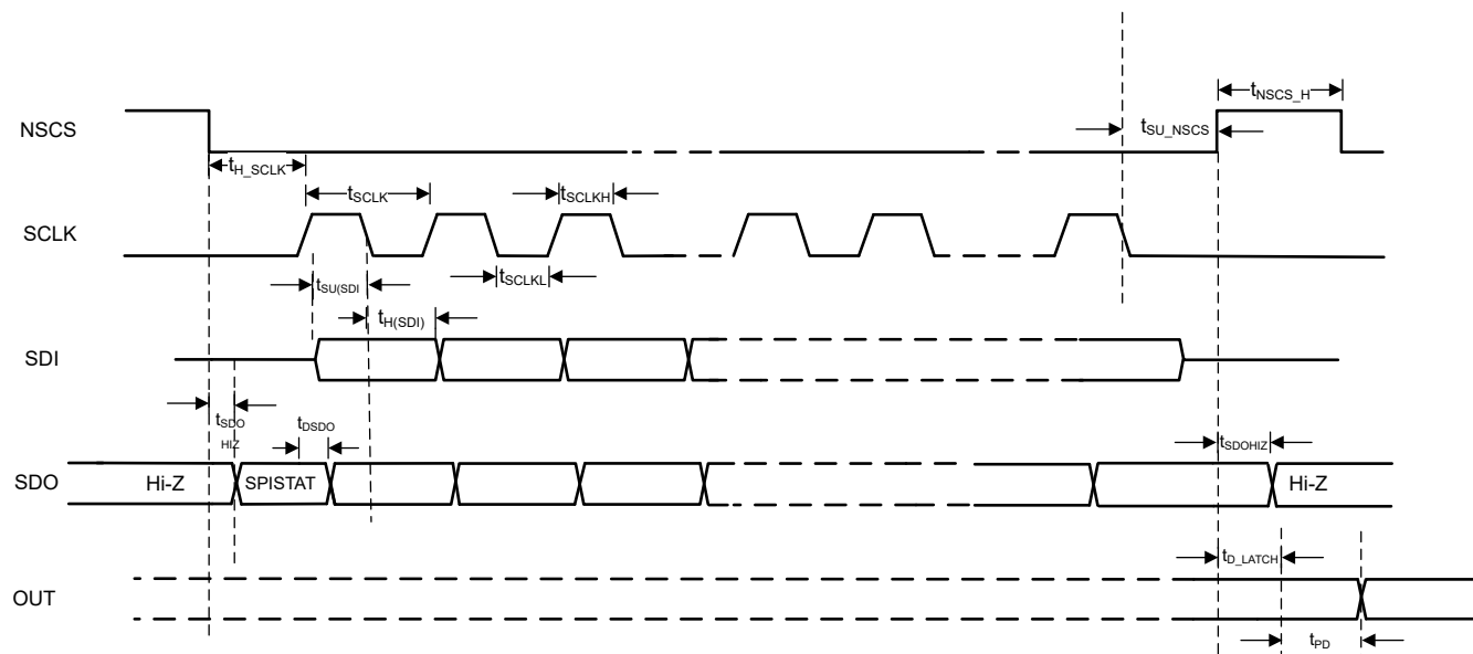
图 5-1. SPI 时序参数
