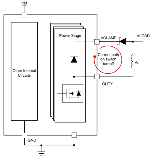
图 6-7. 快速衰减 ( TVS/齐纳二极管 VCLAMP 至 VLOAD )
