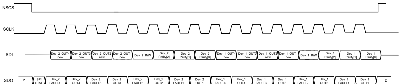
图 6-5. 16 位数据包，用于与两个菊花链器件进行通信
