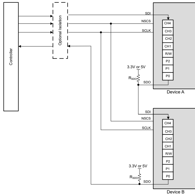
图 6-4. 在菊花链中连接的两个 DRV81646 器件
