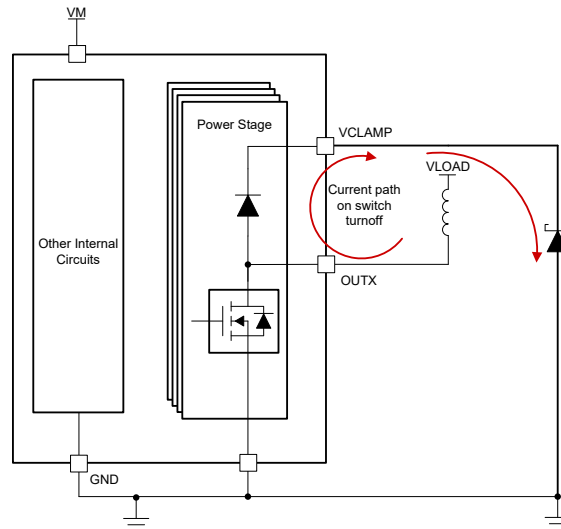
图 6-8. 快速衰减 ( TVS/齐纳钳位至 GND )
