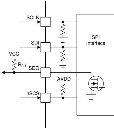
图 8-7. DRV8316CR-Q1 SPI Interface
