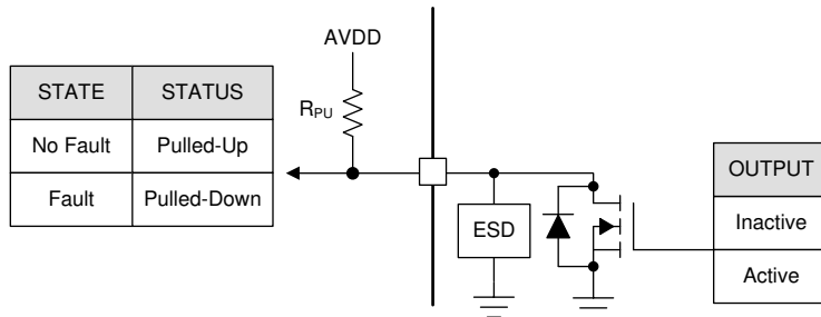
图 8-25. Open Drain
