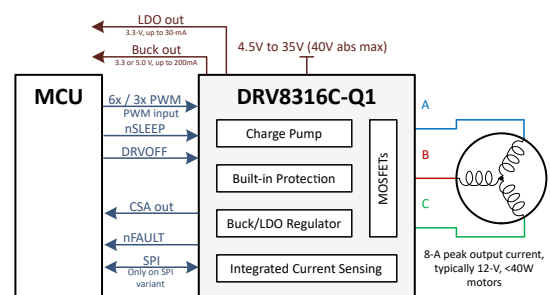
简化原理图
