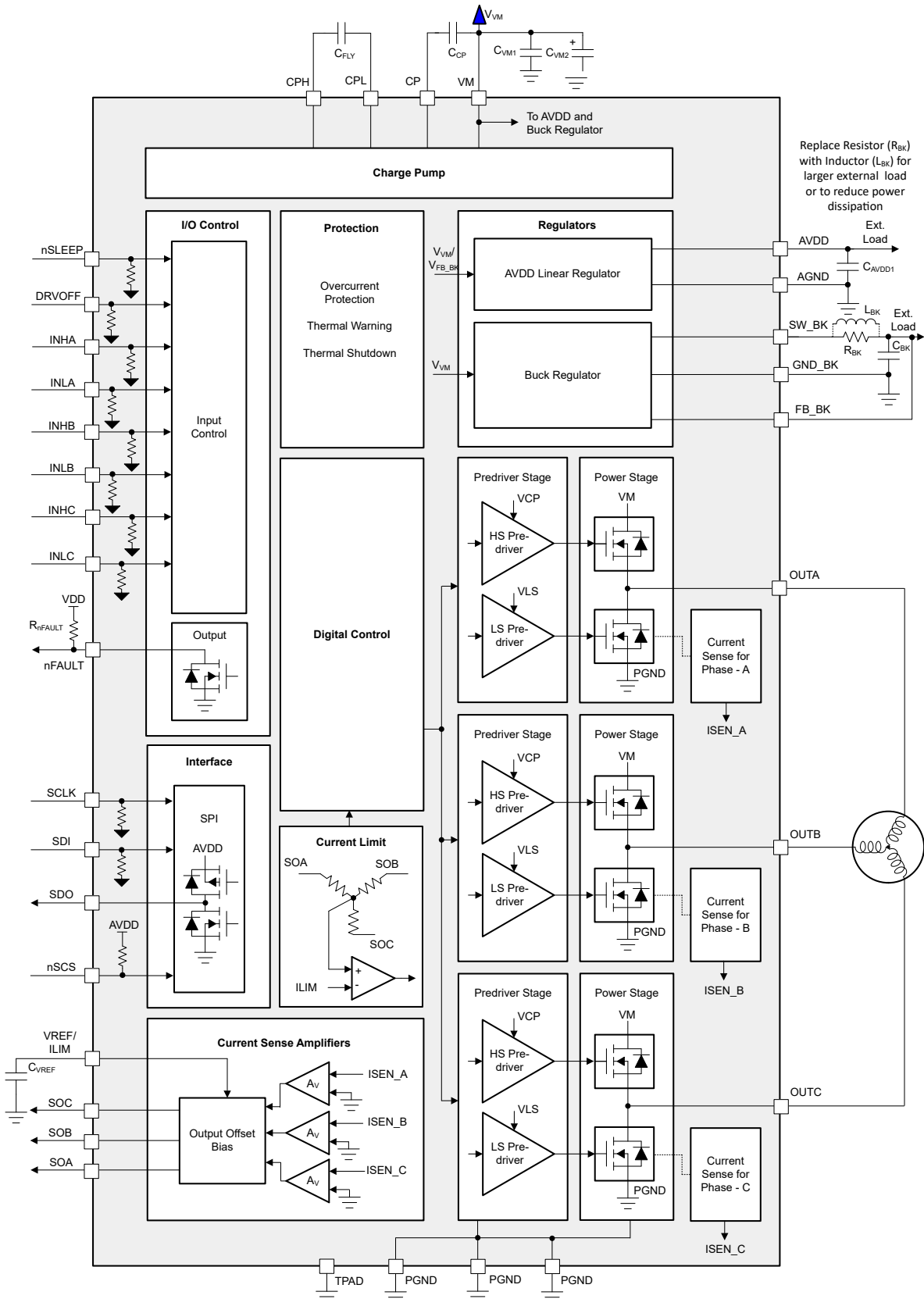
图 8-1. DRV8316C-Q1 Block Diagram
