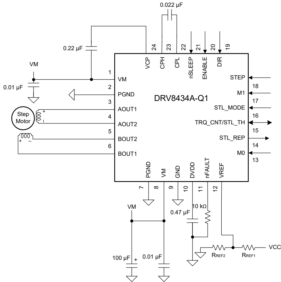
图 7-2. 典型应用原理图
