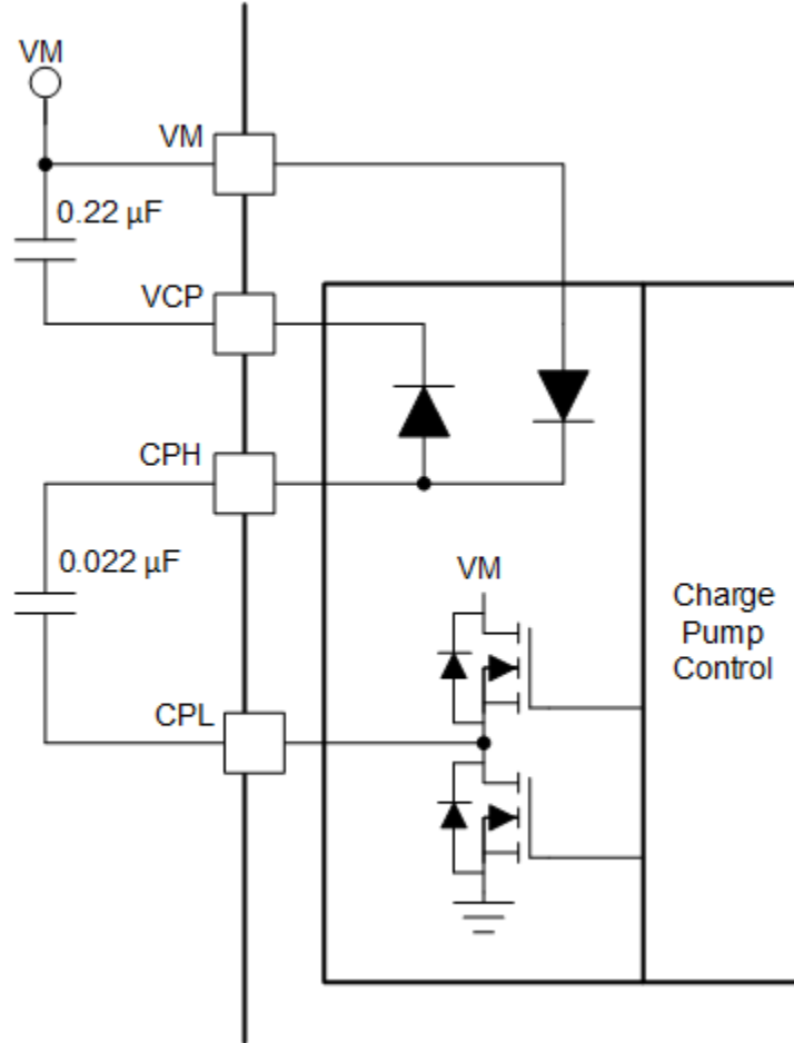
图 6-6. 电荷泵方框图
