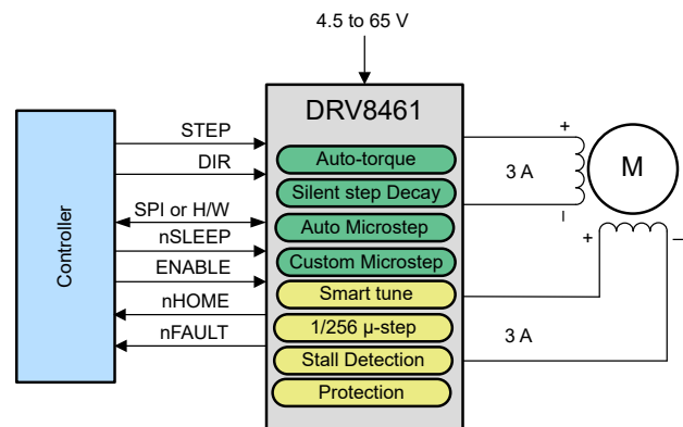
简化原理图
