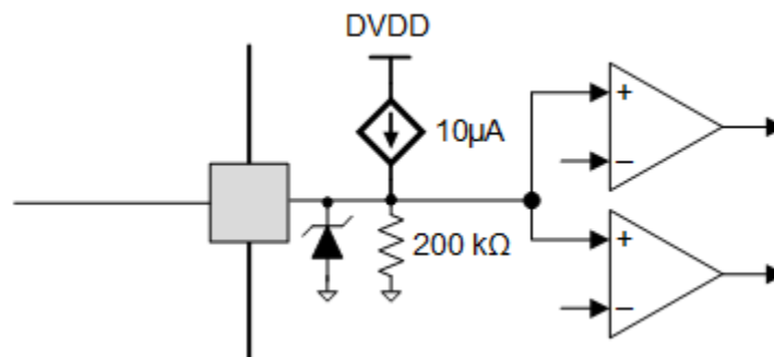
图 7-32. 三电平输入引脚图
