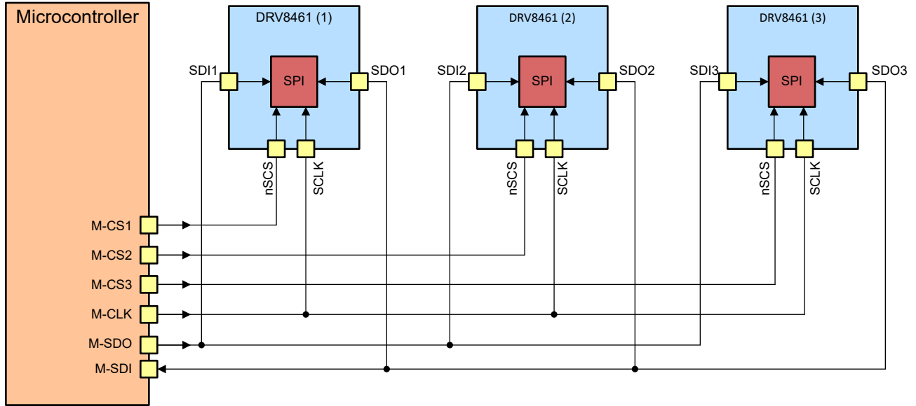
图 7-55. 以并行配置连接的三个器件
