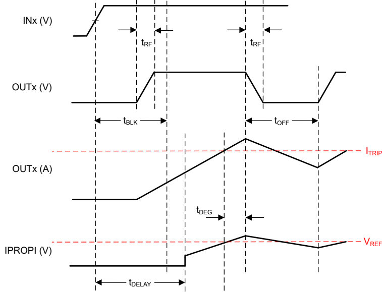
图 6-1. IPROPI 时序图
