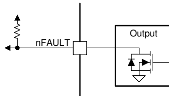
图 7-12. nFAULT 引脚
