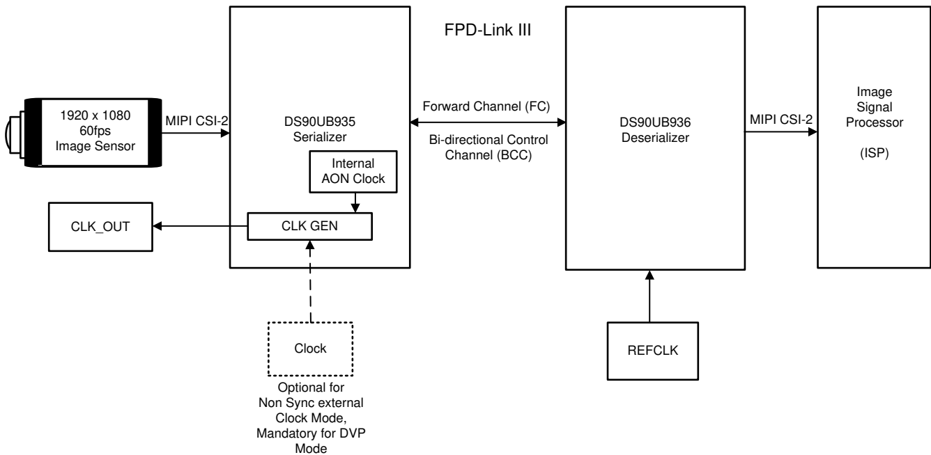
图 6-6. 时钟系统图
