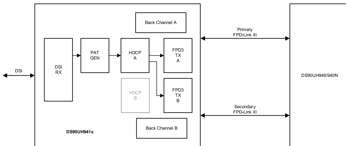
图 8-20. 双链路模式，1:2 模式
