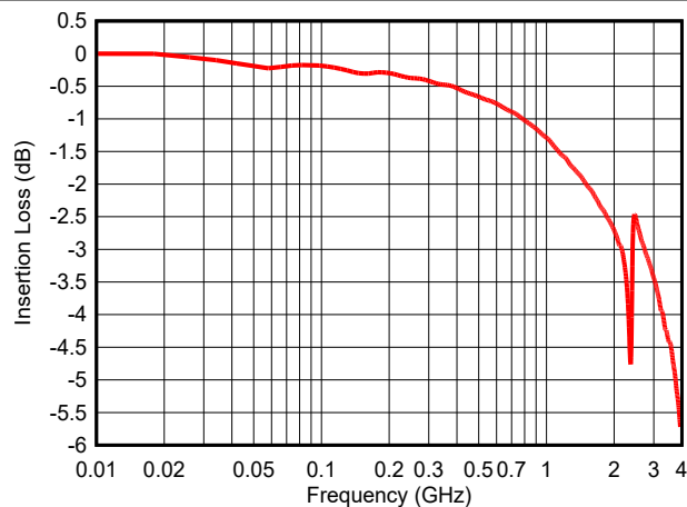
图 5-8. 插入损耗
