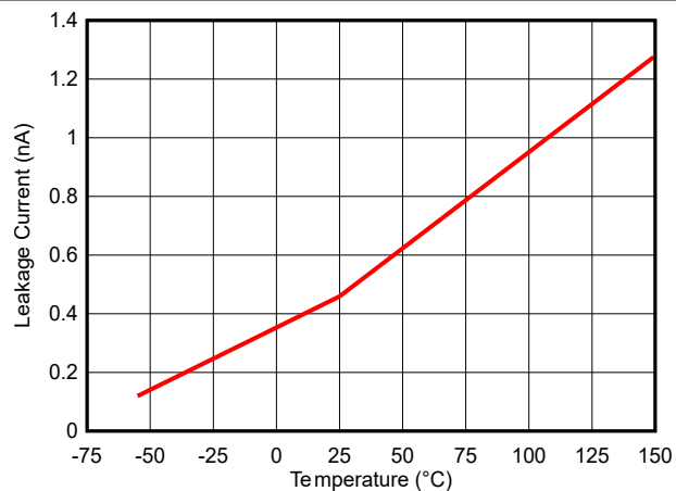
图 5-7. 温度与漏电流间的关系
