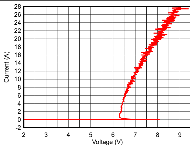
图 5-1. 正 TLP 曲线
