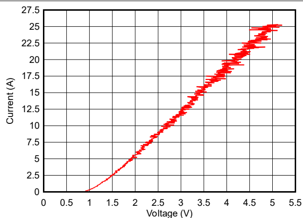
图 5-2. 负 TLP 曲线
