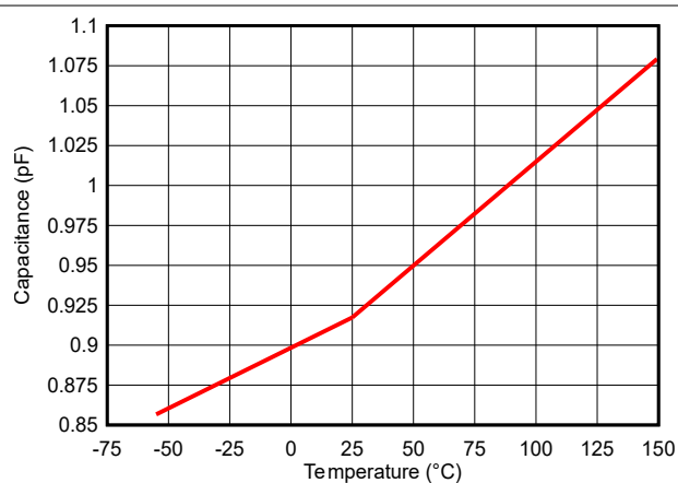
图 5-6. 温度与电容间的关系
