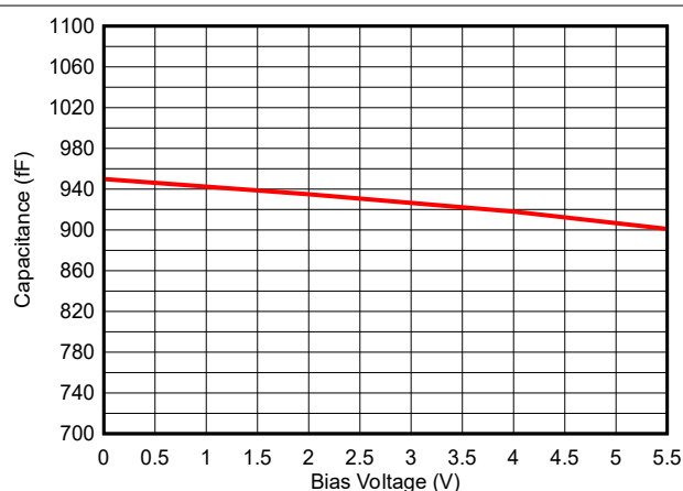
图 5-5. 偏置电压与电容间的关系
