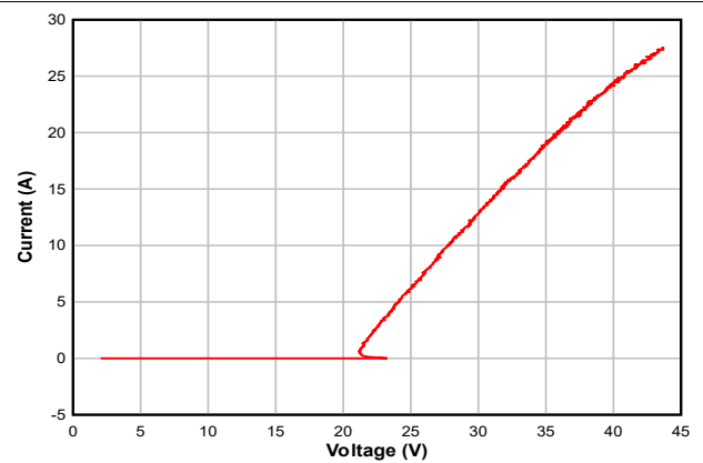
图 5-4. 负 TLP 曲线
