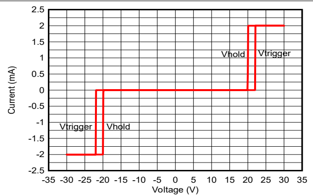
图 5-2. 直流 I-V 曲线
