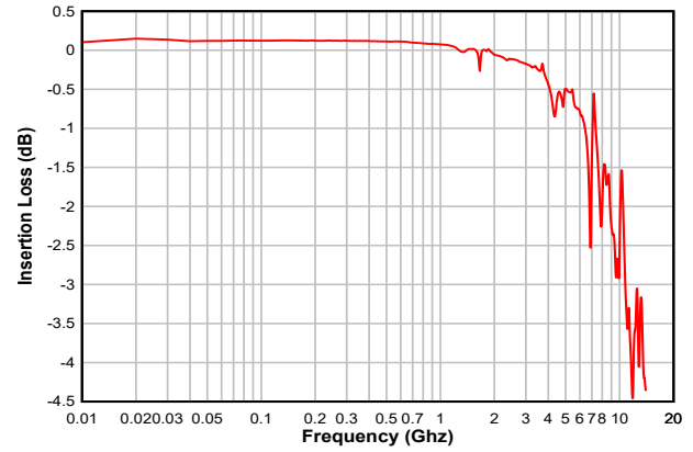
图 5-8. 插入损耗
