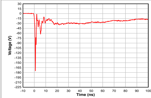
图 5-7. -8kV 钳位 IEC 波形
