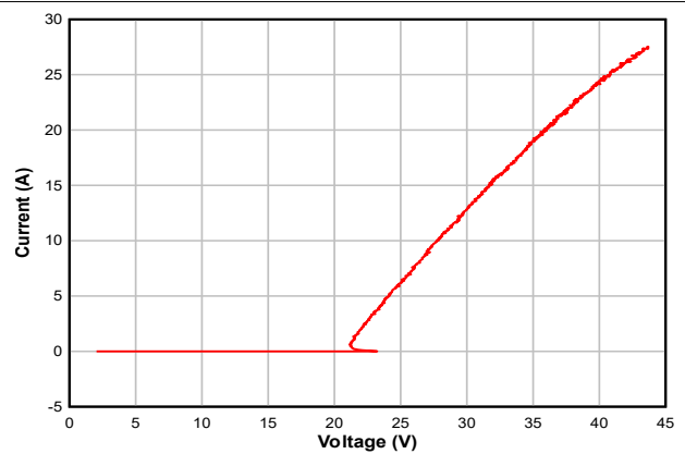
图 5-4. 负 TLP 曲线
