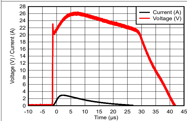
图 5-5. 8/20 \mu s 浪涌响应
