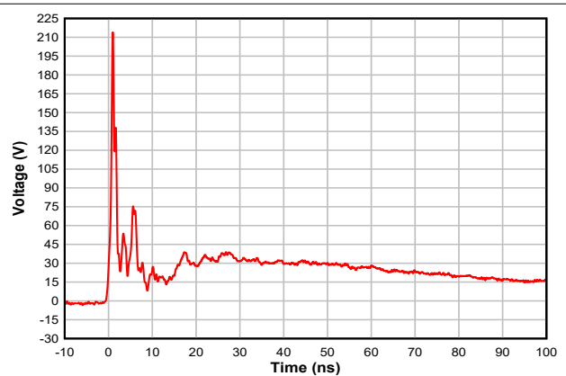
图 5-6. +8kV 钳位 IEC 波形
