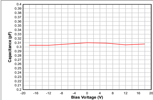
图 5-1. 偏置电压与电容间的关系
