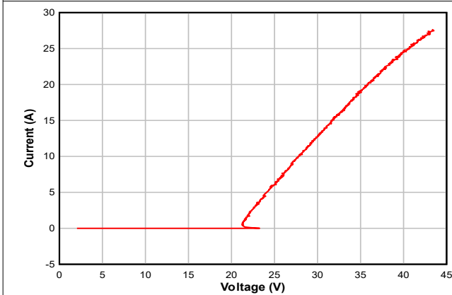
图 5-3. 正 TLP 曲线
