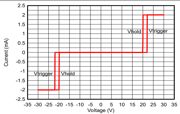
图 5-2. 直流 I-V 曲线
