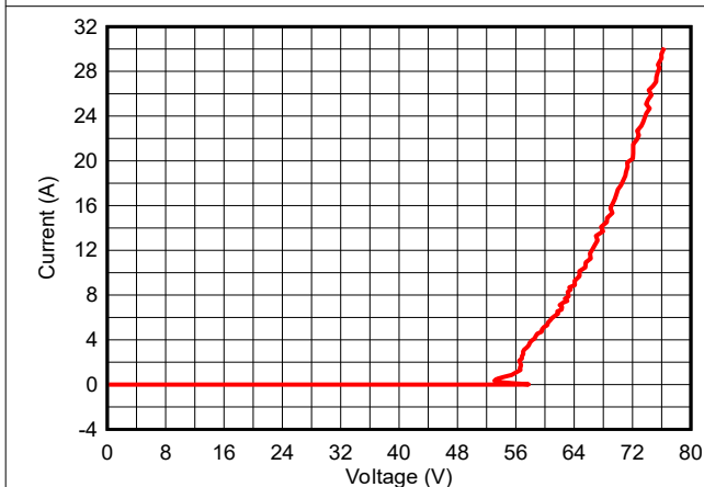
图 5-3. 正 TLP 曲线
