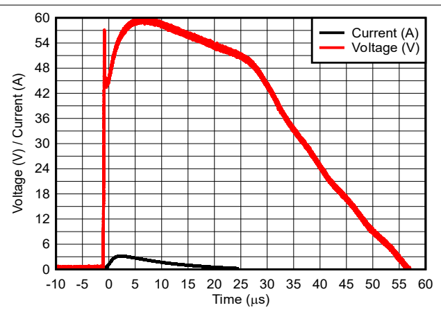
图 5-4. 8/20 μs 浪涌响应
