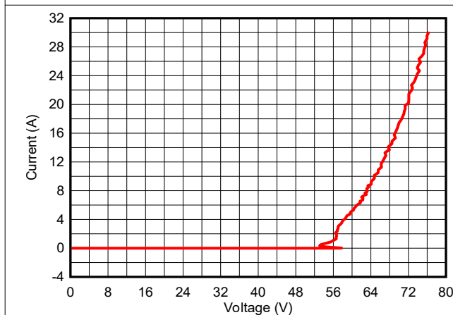
图 5-3. 正 TLP 曲线
