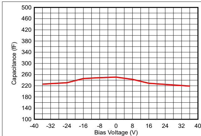
图 5-1. 偏置电压与电容间的关系
