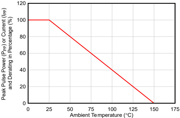
图 5-4. 峰值脉冲功率降额曲线
