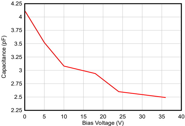
图 5-2. 电容与偏置电压之间的关系
