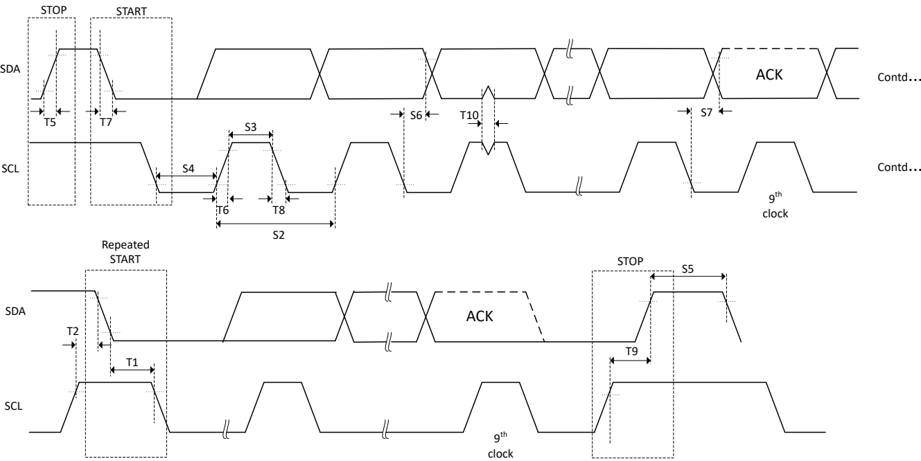
图 6-83. I2C 时序图
