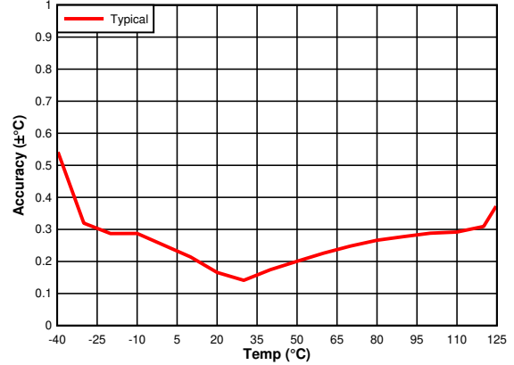
图 6-3. 温度精度与温度设定点间的关系
