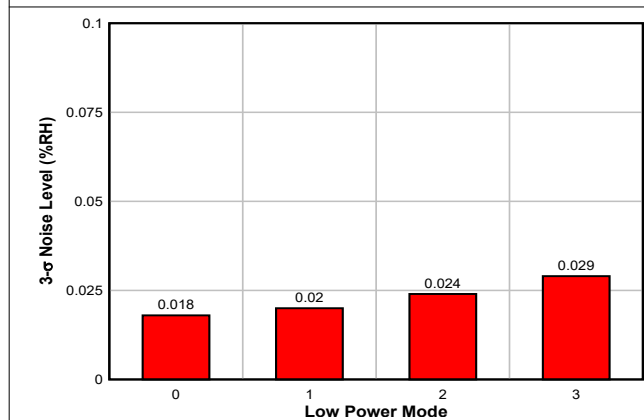
图 6-6. 低功耗模式下的典型 RH 噪声
