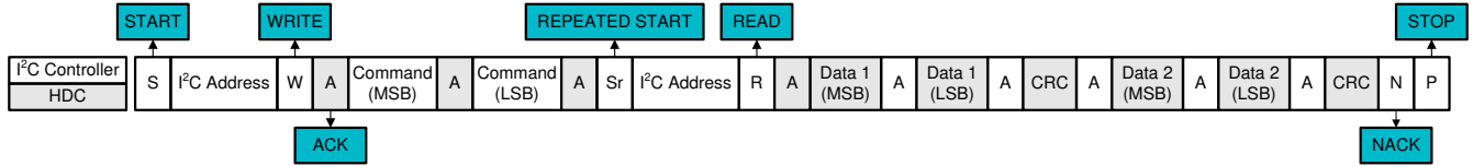
图 7-6. I 2 C 重复启动序列，多个数据结果
