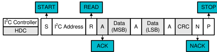
图 7-3. I 2 C 读取单个数据结果
