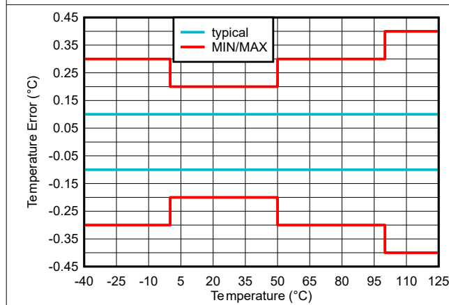
图 6-4. 温度精度与温度间的关系
