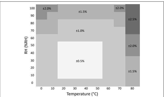
图 6-3. 相对湿度和温度范围内的典型 RH 精度
