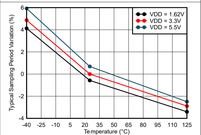
图 6-5. 自动采样时序变化
