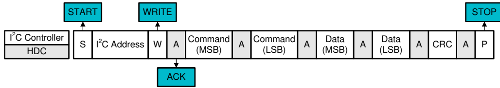
图 7-2. 需要 I 2 C 写入命令、配置数据和 CRC 字节
