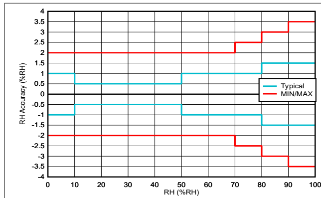
图 6-2. RH 精度与 RH 间的关系
