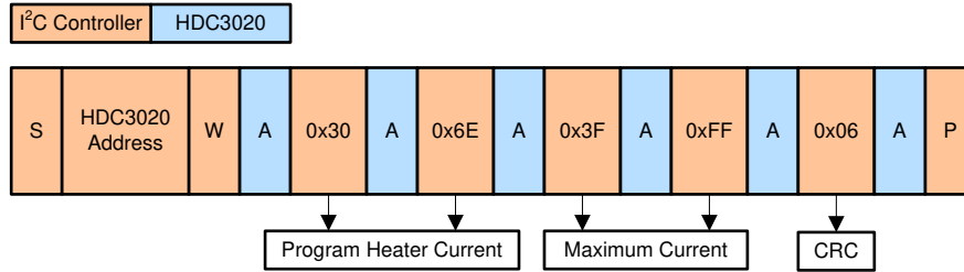
图 7-28. I 2 C 命令序列：配置加热器电流全功率
