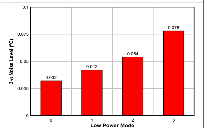
图 6-7. 低功耗模式下的典型温度噪声
