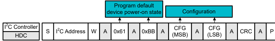
图 7-15. I 2 C 序列：配置默认上电状态和采样周期
