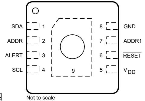
图 5-1. HDC302x-Q1 DEF、DEH、DEJ 封装 8 引脚 WSON 透明顶视图
