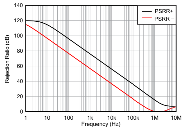
图 7-26. PSRR 与频率间的关系 (RTI)
