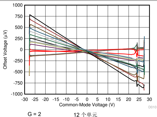
图 7-10. 失调电压与共模电压间的关系
