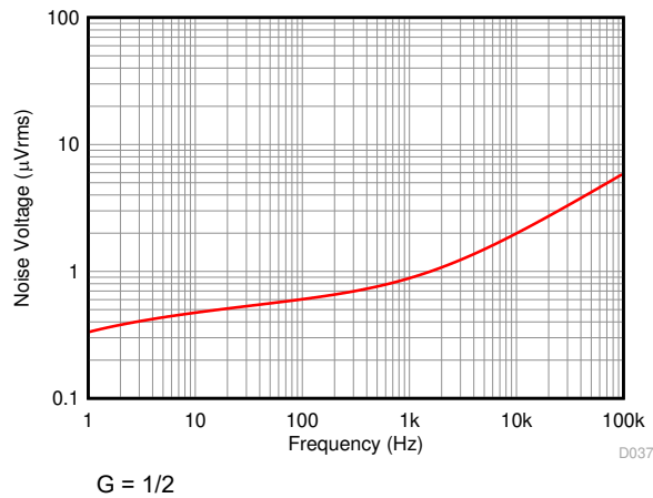
图 7-37. 集成输出电压噪声与噪声带宽间的关系
