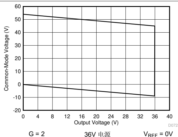
图 7-72. 输入共模电压与输出电压间的关系
