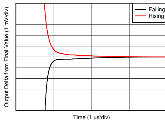
图 7-44. 建立时间
