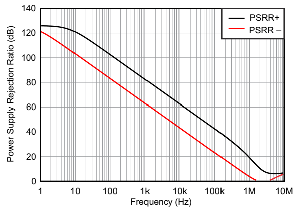
图 7-25. PSRR 与频率间的关系 (RTI)
