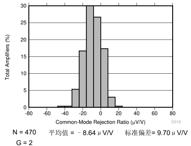
图 7-18. 典型 CMRR 分布
