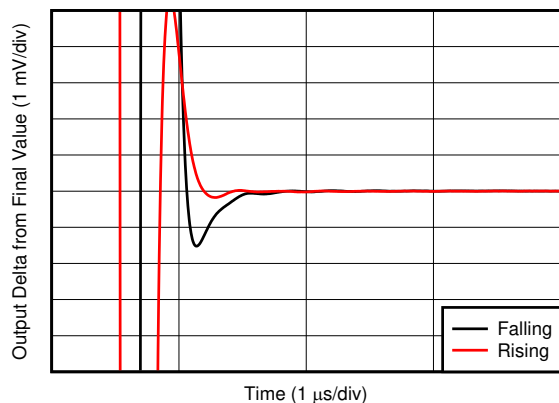
图 7-43. 建立时间
