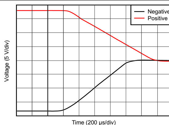
图 7-46. 大信号阶跃响应
