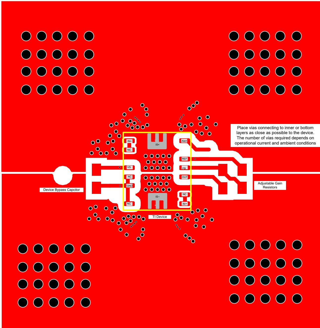
图 7-10. INA751x-Q1 布局示例
