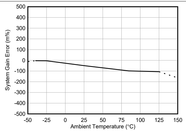
图 5-14. INA751B-Q1 增益误差与温度间的关系
