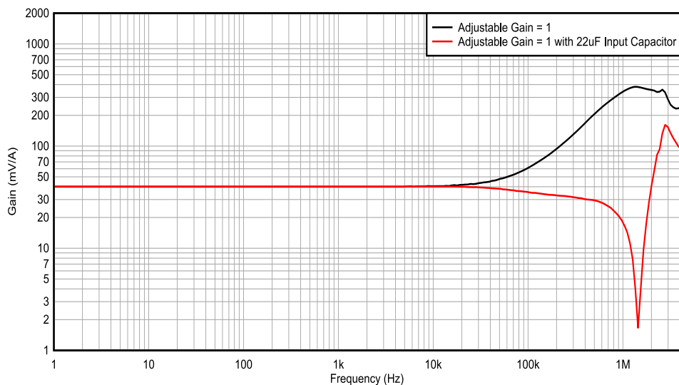
图 7-4. 添加 22 \mu F 输入电容器之前和之后 INA751x-Q1 增益与频率间的关系
