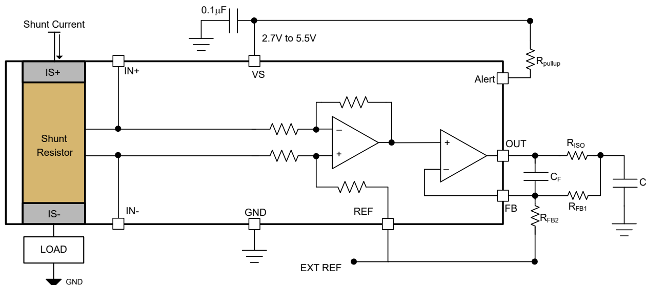
图 7-5. 具有 RISO 双反馈的 INA751x-Q1
