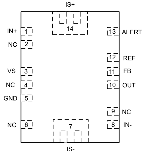
图 4-1. INA751x-Q1 REM 封装 VQFN 顶视图
