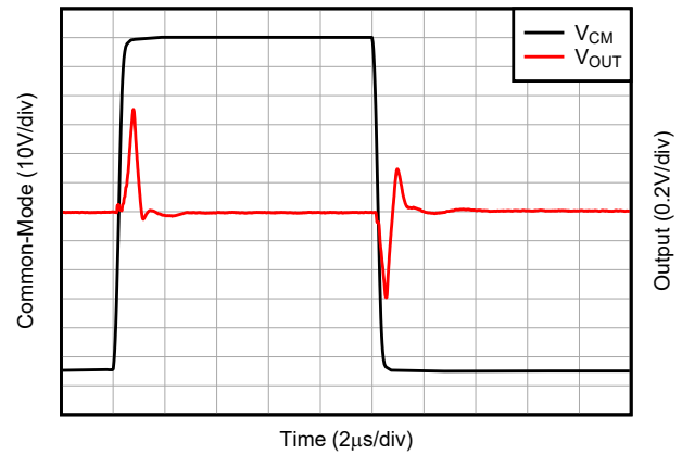
图 5-34. 共模瞬态响应
