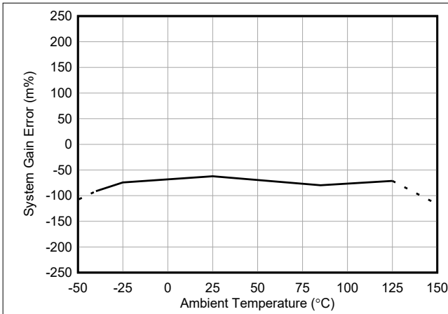
图 5-13. INA751A-Q1 增益误差与温度间的关系
