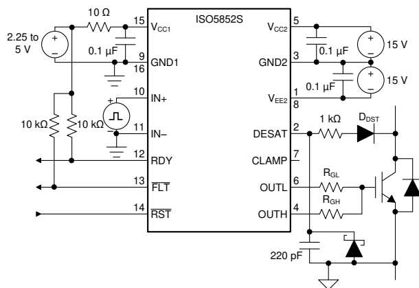
图 10-3. Bipolar Output Supply
