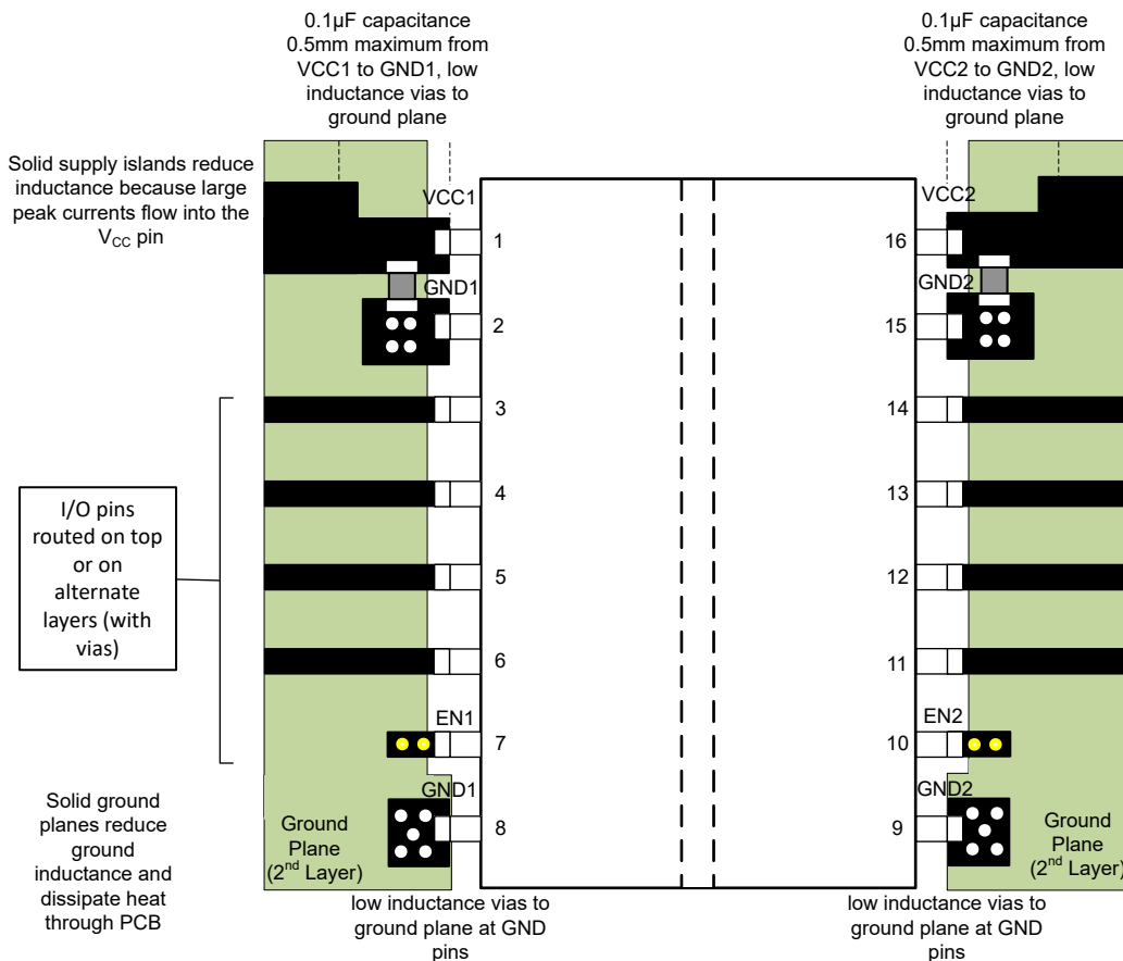
图 9-6. 布局示例
