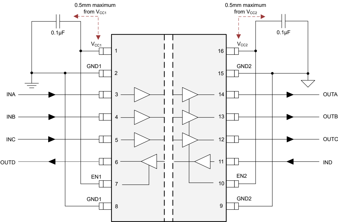
图 9-2. 典型 ISO644x 电路
