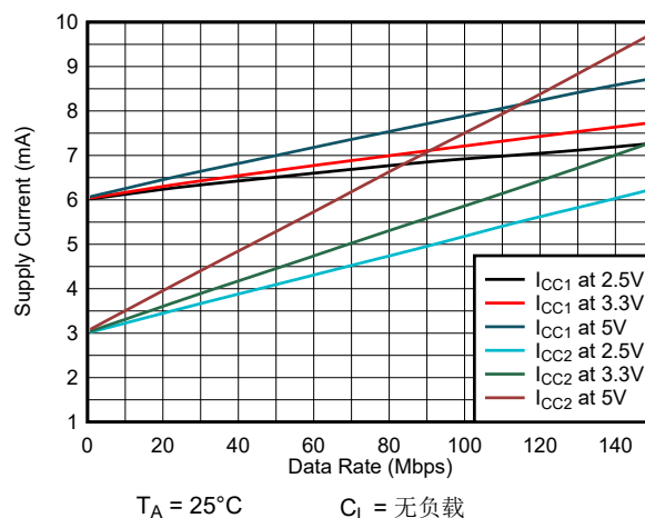
图 6-10. ISO6441 或 ISO6441F 电源电流与数据速率间的关系 (无负载)
