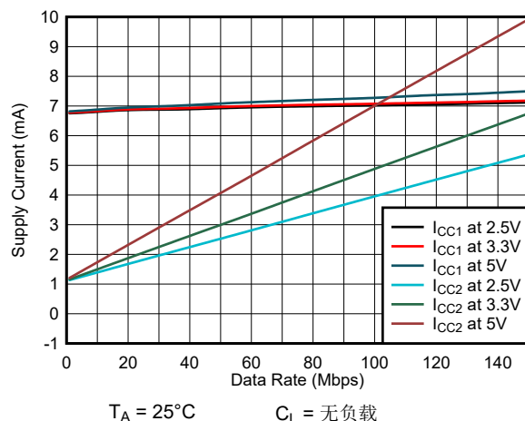
图 6-8. ISO6440 或 ISO6440F 电源电流与数据速率间的关系 (无负载)
