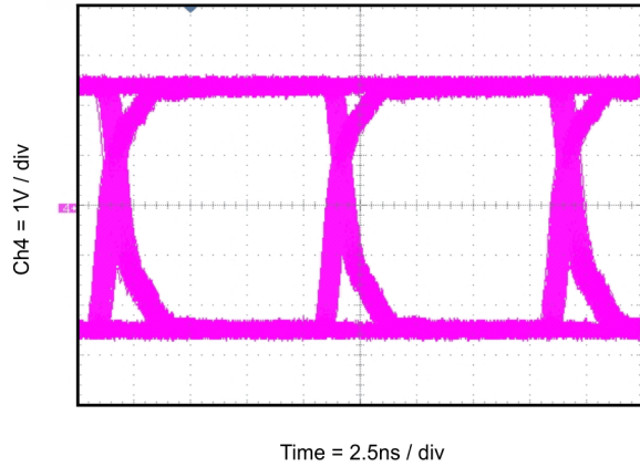
图 8-4. 眼图：100Mbps PRBS 2^{16} - 1 ，5V，25°C
