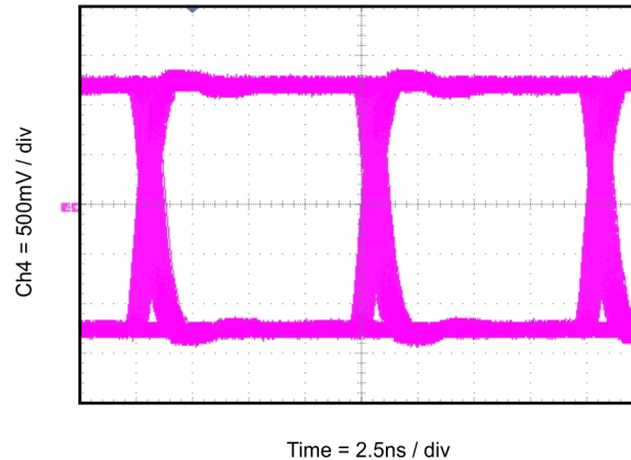
图 8-6. 眼图：100Mbps PRBS 2^{16} - 1 ，2.5V，25°C
