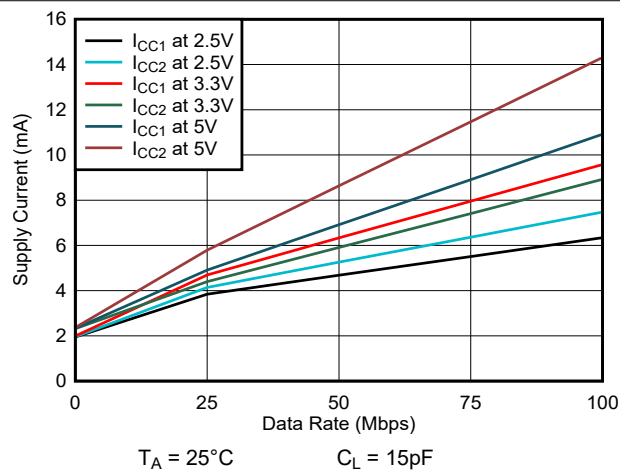
图 5-7. ISO7731 电源电流与数据速率间的关系 (具有 15pF 负载)
