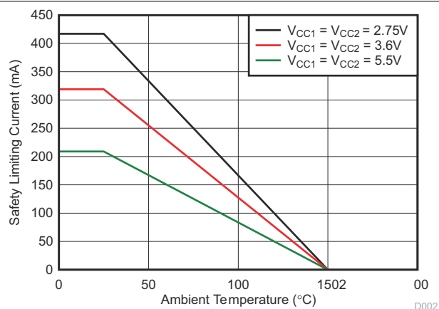
图 5-2. DBQ-16 封装根据 VDE 标准安全限制电流的热降额曲线
