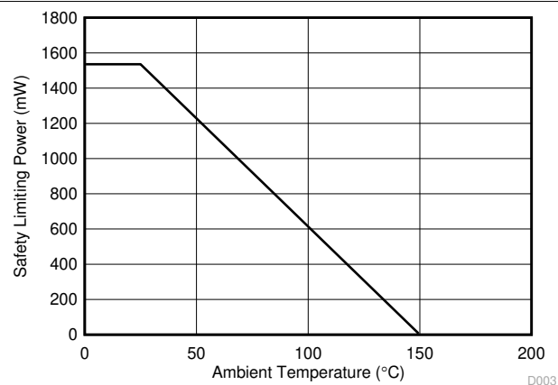
图 5-3. DW-16 封装根据 VDE 标准安全限制功率的热降额曲线
