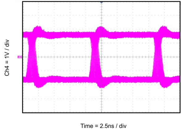
图 8-5. 眼图：100Mbps PRBS 2^{16} - 1 ，3.3V，25°C
