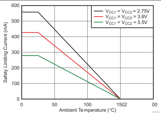
图 5-1. DW-16 封装根据 VDE 标准安全限制电流的热降额曲线
