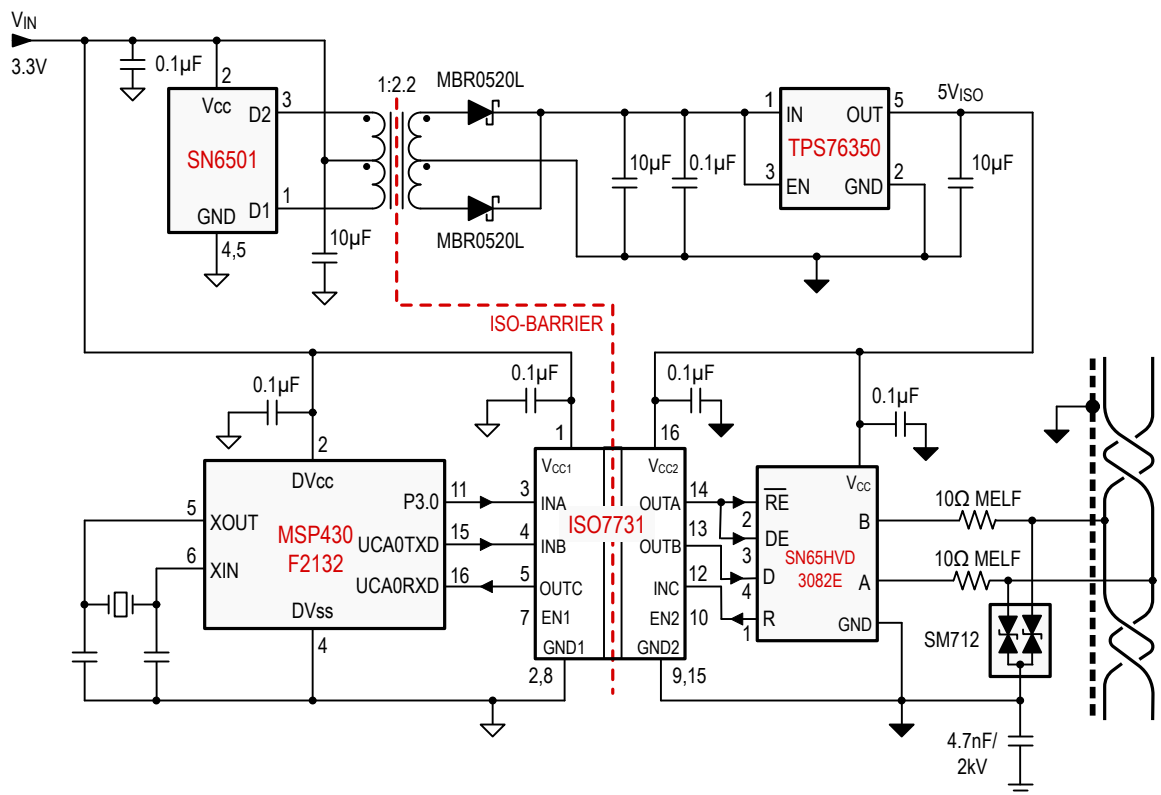
图 8-1. 隔离式 RS-485 接口线路
