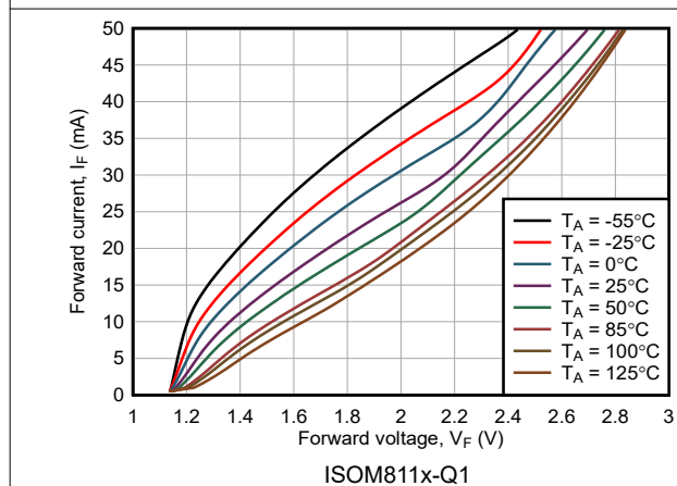
图 6-3. 正向电压与正向电流间的关系
