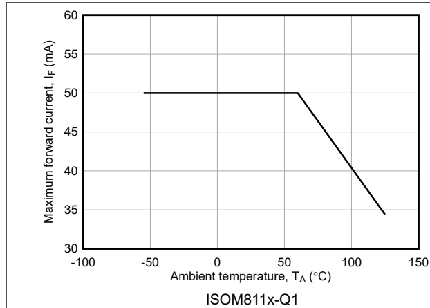
图 6-1. 最高正向电流与环境温度间的关系
