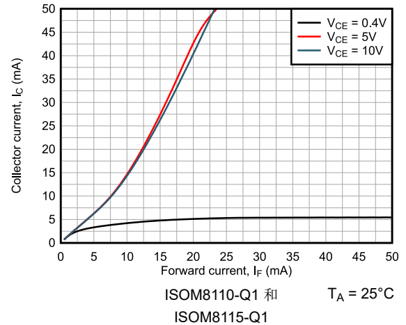
图 6-10. 集电极电流与正向电流间的关系
