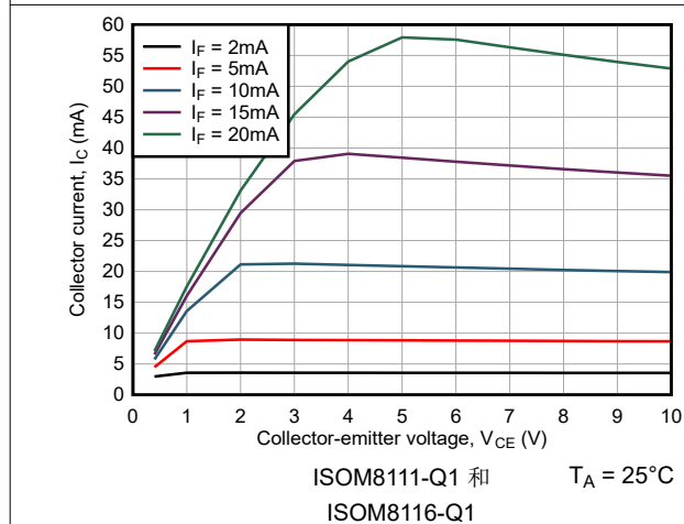
图 6-5. 集电极电流与集电极-发射极电压间的关系
