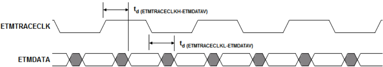
图 7-17. ETMDATA 时序
