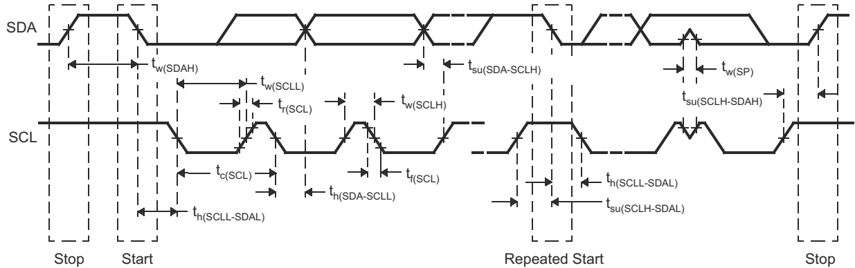
图 7-19. I2C 时序图
