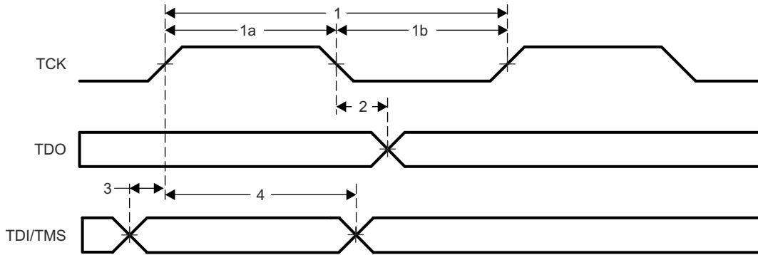
图 7-22. JTAG 时序
