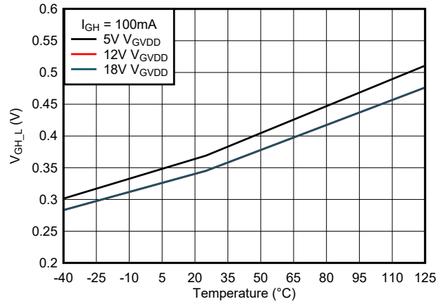
图 6-11. GH Output Low Voltage vs Temperature
