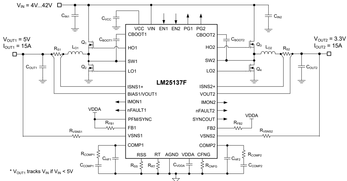
LM25137F 双路输出降压开关稳压器 - 简化原理图
