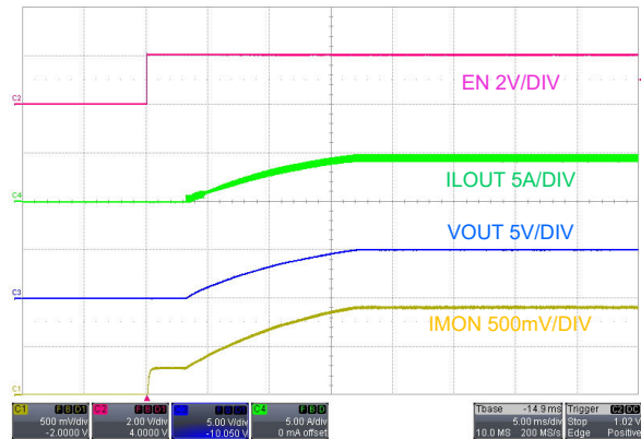
图 7-7. 启动，EN 开启， V_{SUPPLY} = 12V ， I_{LOAD} = 5A 电阻负载
