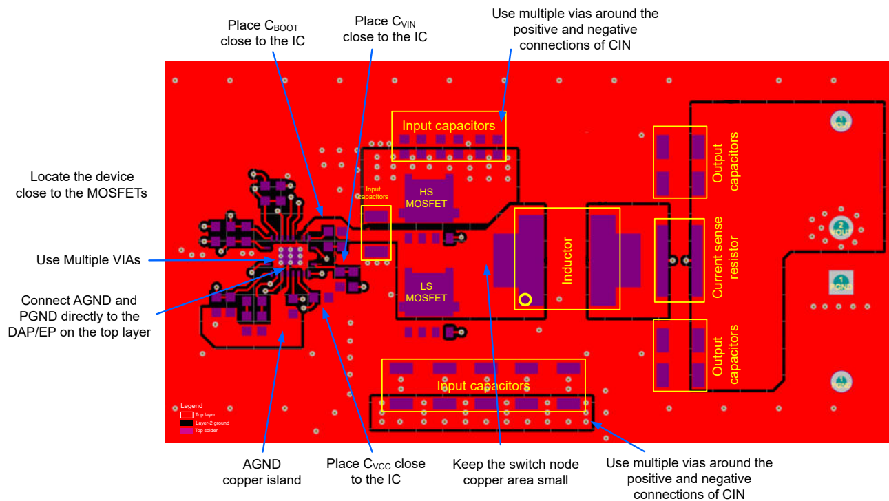
图 10-12. PCB 顶层
