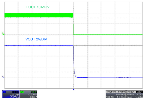
图 10-6. 关断，EN 关闭， V_{\text{SUPPLY}} = 12\text{V} ， I_{\text{LOAD}} = 18\text{A} 电阻负载
