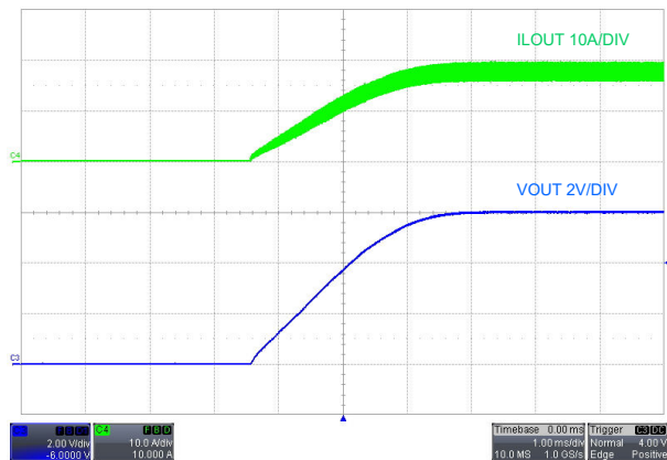
图 10-5. 启动，EN 开启， V_{\text{SUPPLY}} = 12\text{V} ， I_{\text{LOAD}} = 18\text{A} 电阻负载
