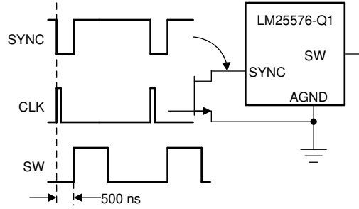
图 6-3. 与外部时钟同步
