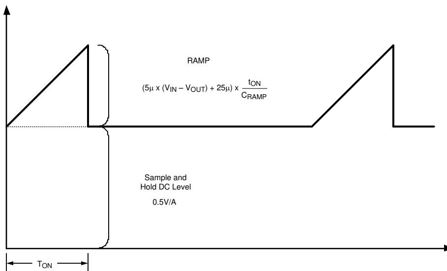
图 6-6. 电流检测信号的组成
