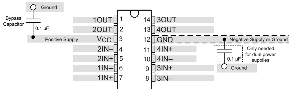
图 9-4. LMx39 Layout Example
