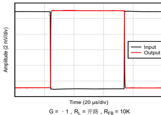
图 5-27. 小信号阶跃响应, G = -1
