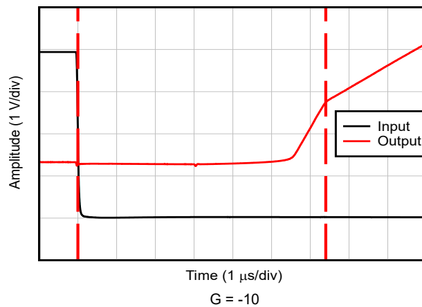
图 5-25. 过载恢复 (负轨)
