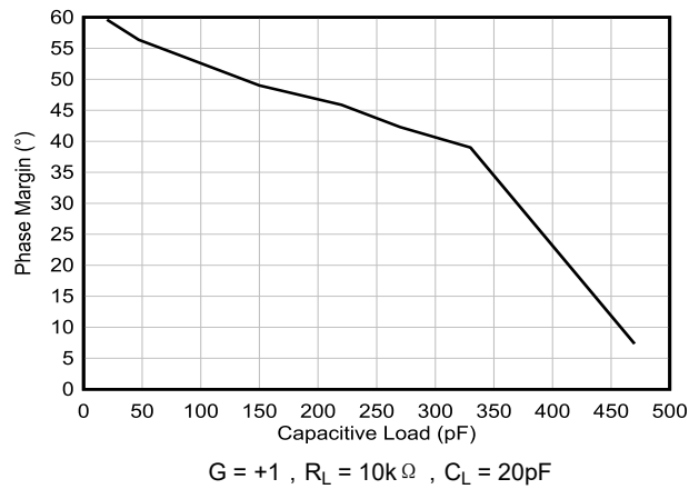
图 5-23. 相位裕度与容性负载间的关系
