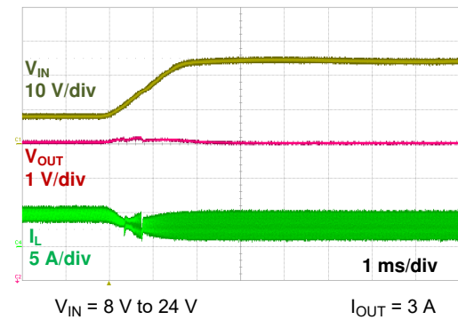
图 6-18. Line Transient
