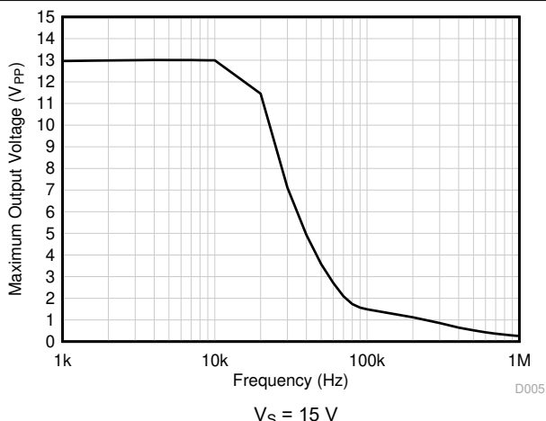
图 5-36. 最大输出电压与频率间的关系
