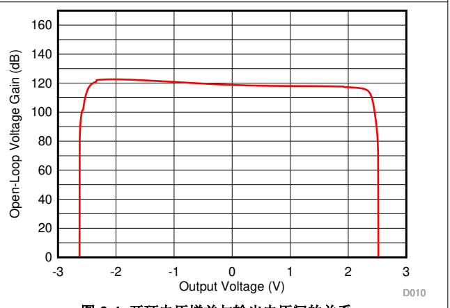
图 6-4. 开环电压增益与输出电压间的关系
