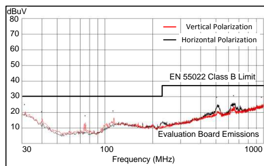
辐射发射图
