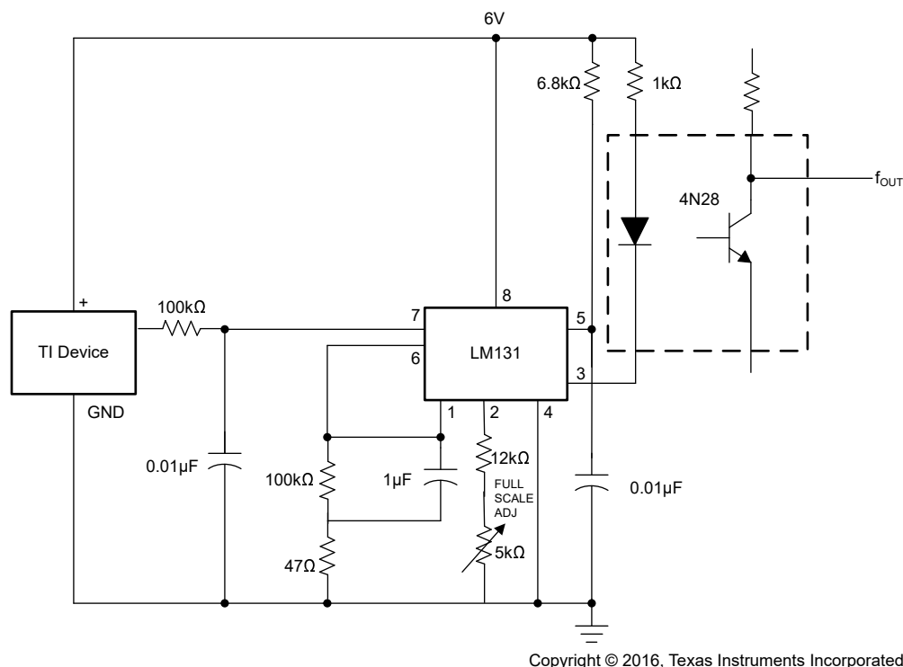
图 8-12. 具有压频转换器和隔离式输出的 LM50 和 LM50HV
