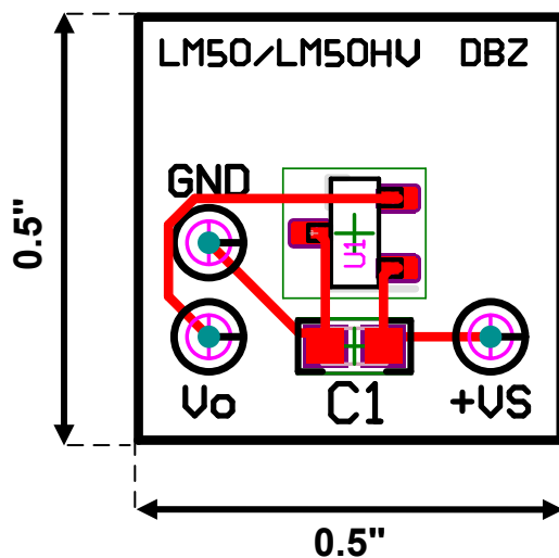
图 8-15. 用于生成热响应曲线的印刷电路板 [LM50 (新芯片和旧芯片) 和 LM50HV 的新测试设置]
