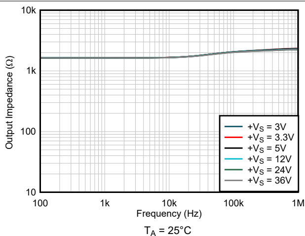
图 6-33. 输出阻抗与频率间的关系
