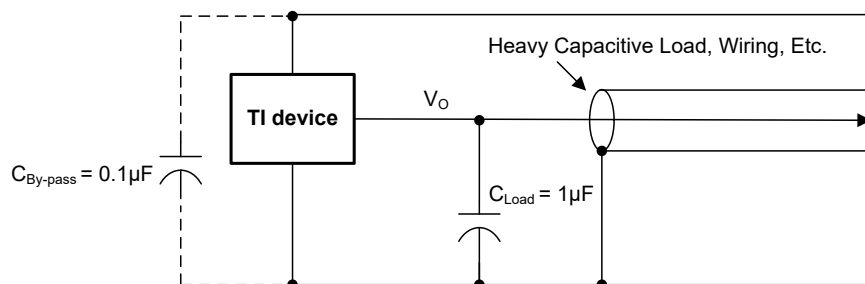
图 8-3. 具有滤波器且适用于噪声环境的 LM50 和 LM50HV
