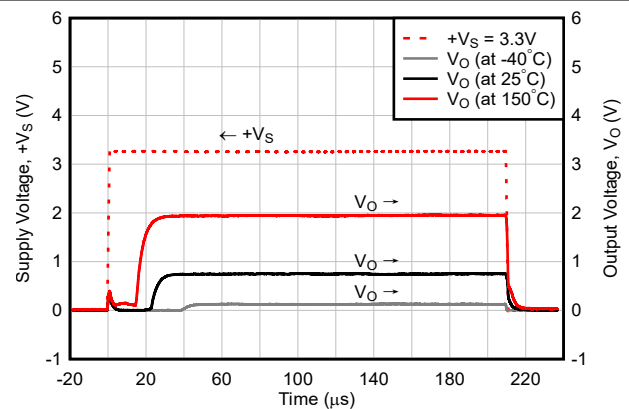
图 6-30. +V_S = 3.3\text{V} 阶跃时的启动响应 (当 t_r = 1\text{ }\mu\text{s} 、无 C_{\text{Load}} 和 C_{\text{By-pass}} 时)
