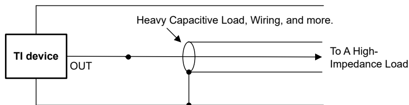
图 8-2. LM50 和 LM50HV 电容负载无需去耦
