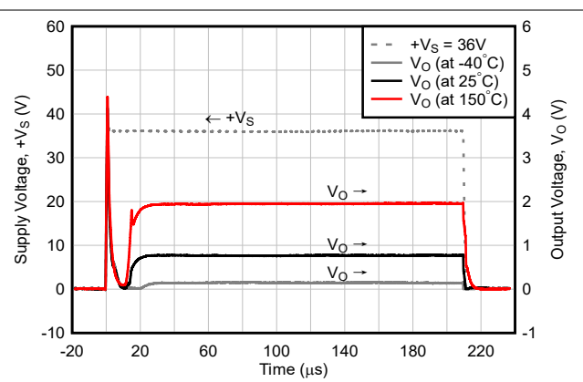
图 8-5. +V_S = 36V 阶跃时的启动响应（当 t_r = 1\mu s ，无 C_{Load} 和 C_{By-pass} 时）
