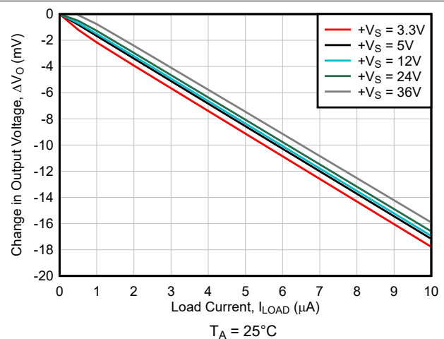
图 6-28. 输出电压与负载电流变化间的关系
